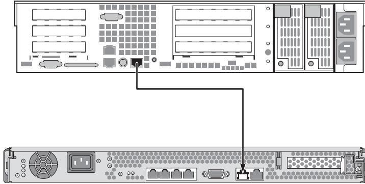
FIGURE 1-4 Connexion TIP entre un serveur et un autre système Sun
