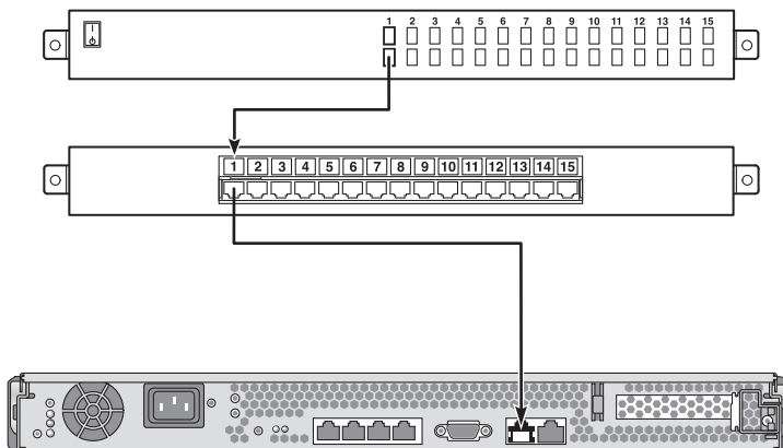
FIGURE 1-3 Connexion d'un serveur de terminaux à un serveur au moyen d'un tableau de connexions
