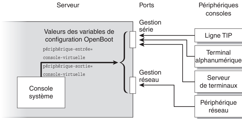
FIGURE 1-1 Redirection de la console système
