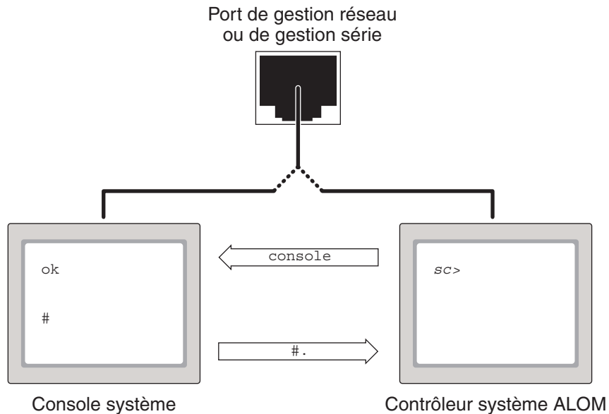
FIGURE 1-5 Basculement entre la console système et l'invite du contrôleur système
