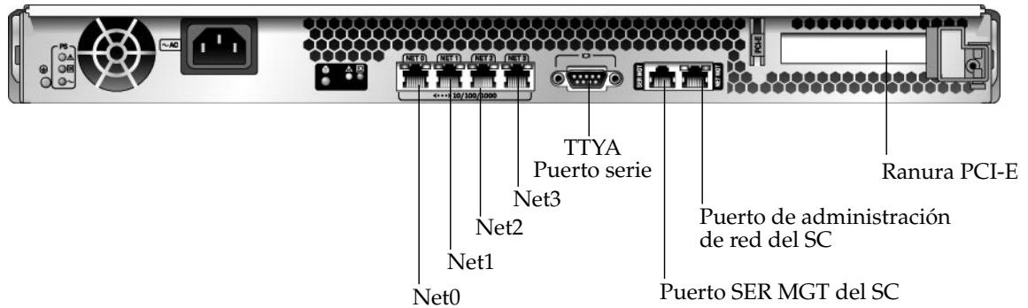
FIGURA 1-2 Panel de E/S trasero del chasis
