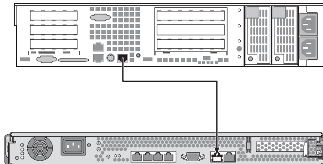
그림 1-4 서버와 다른 Sun 시스템 간 TIP 연결
