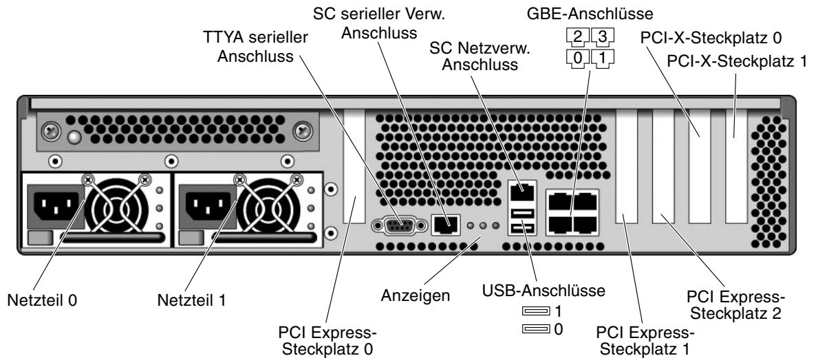
ABBILDUNG 4 Rückseite des Sun SPARC Enterprise T2000-Servers
