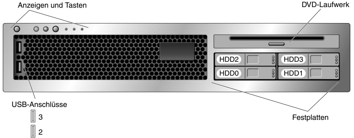
ABBILDUNG 3 Vorderseite des Sun SPARC Enterprise T2000-Servers
