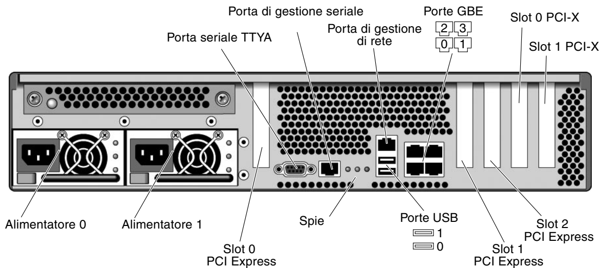
FIGURA 4 Pannello posteriore del server Sun SPARC Enterprise T2000
