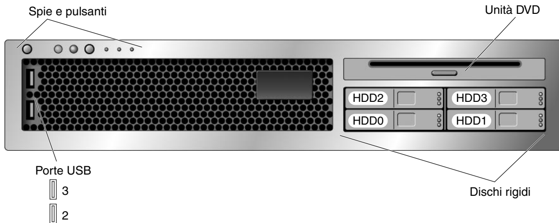
FIGURA 3 Pannello anteriore del server Sun SPARC Enterprise T2000
