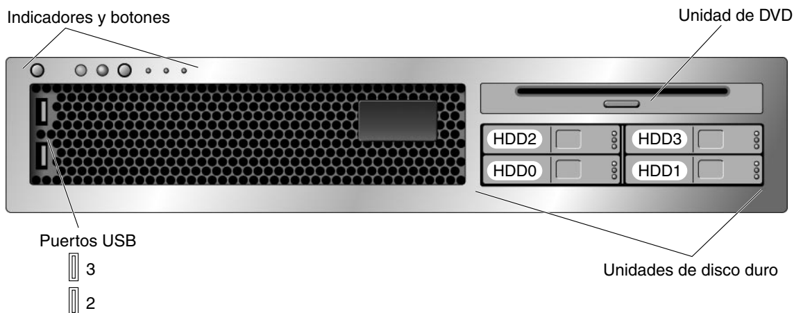
FIGURA 3 Panel frontal del servidor Sun SPARC Enterprise T2000
