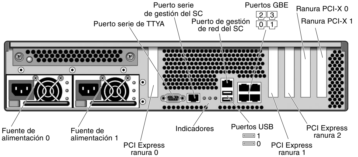
FIGURA 4 Panel posterior del servidor Sun SPARC Enterprise T2000
