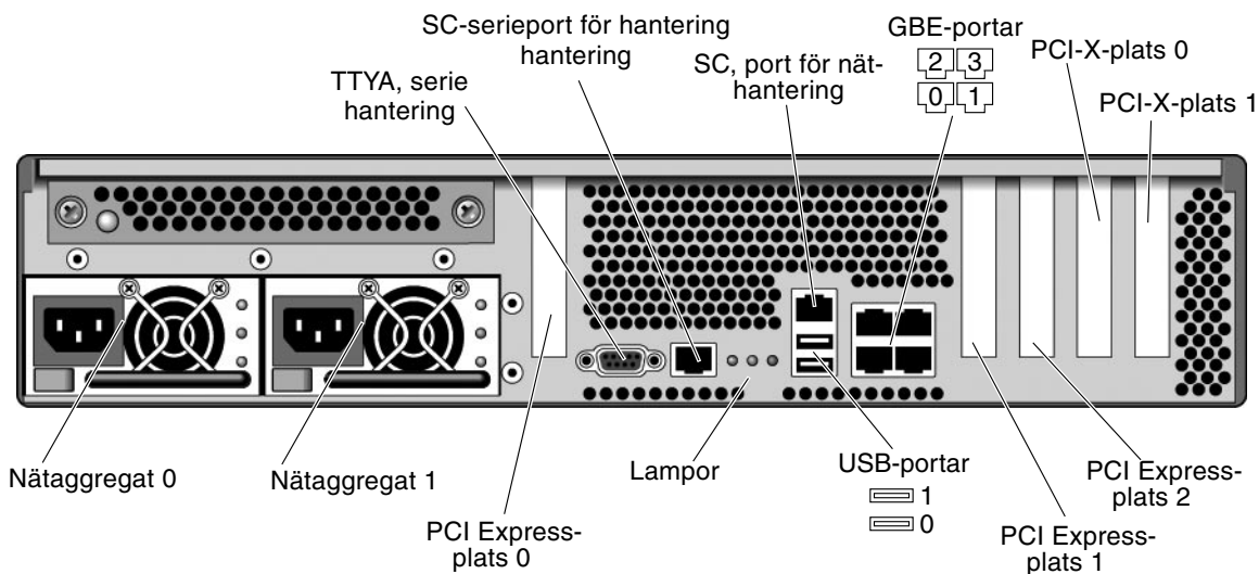
FIGUR 4 Bakpanelen på Sun SPARC Enterprise T2000
