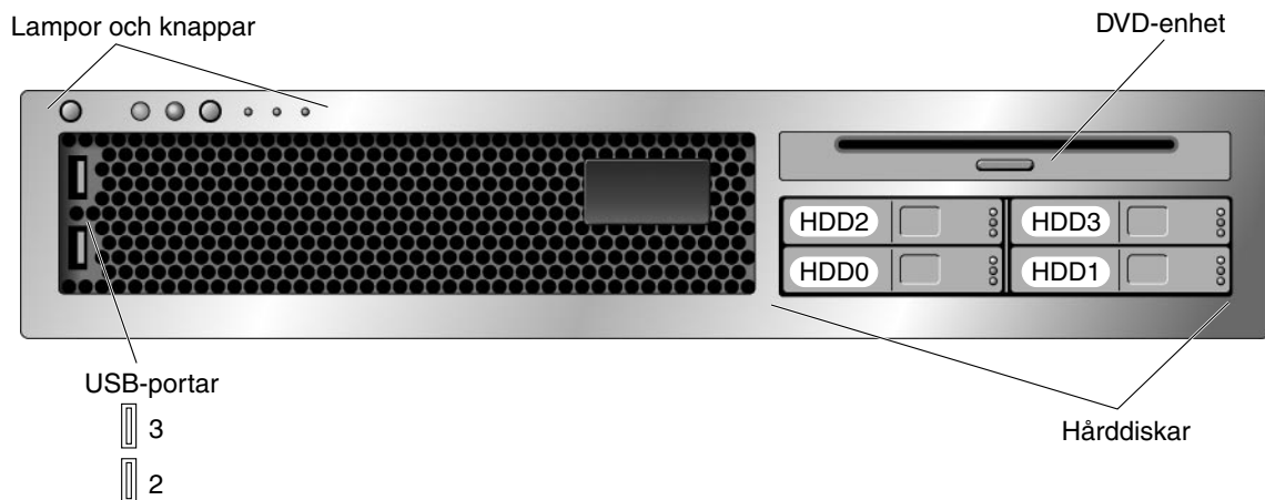
FIGUR 3 Framsidan på Sun SPARC Enterprise T2000
