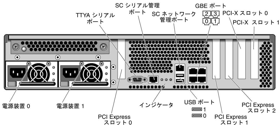
図 4 Sun SPARC Enterprise T2000 サーバの背面パネル
