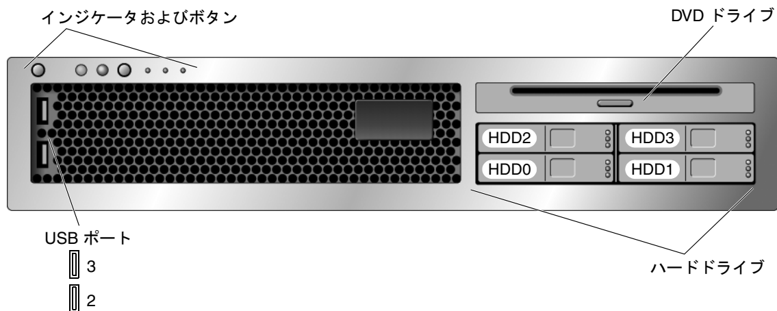
図 3 Sun SPARC Enterprise T2000 サーバのフロントパネル
