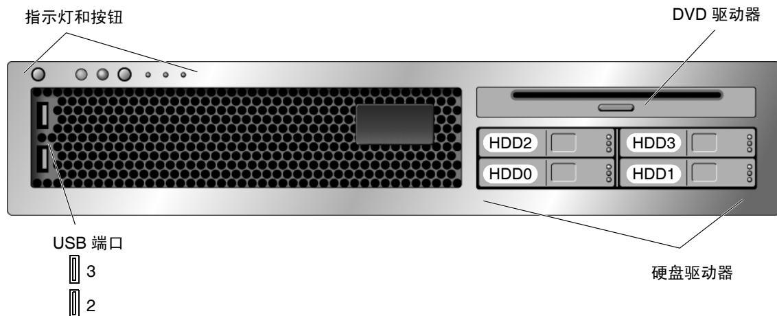
图 3 Sun SPARC Enterprise T2000 服务器前面板
