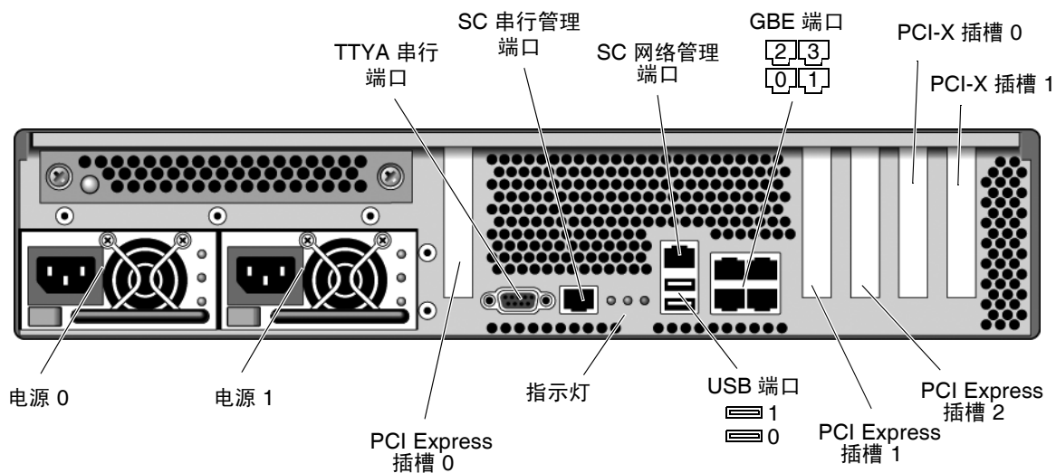
图 4 Sun SPARC Enterprise T2000 服务器后面板
