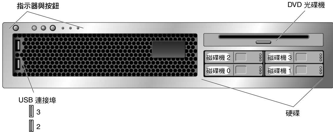
圖 3 Sun SPARC Enterprise T2000 伺服器前方面板
