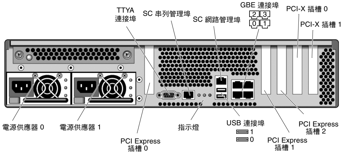
圖 4 Sun SPARC Enterprise T2000 伺服器後方面板
