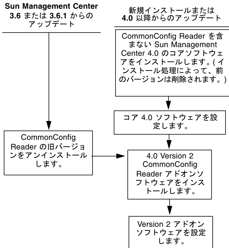
図 1 インストール処理の流れ
