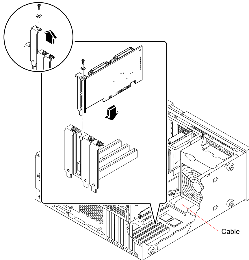
FIGURA 1-4 Ranuras PCI del sistema Ultra 60
