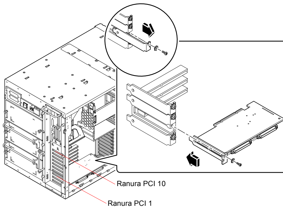
FIGURA 1-8 Ranuras PCI del sistema Sun Enterprise 450
