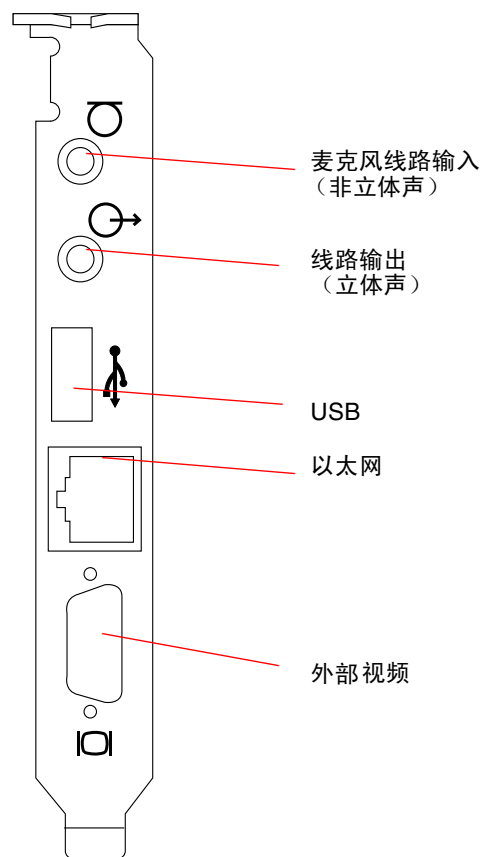
图 10-1 SunPCi II 卡挡板接口
