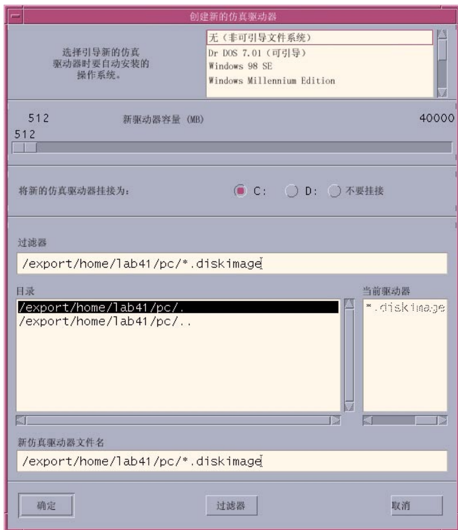
图 2-2 “创建新的仿真驱动器”对话框
