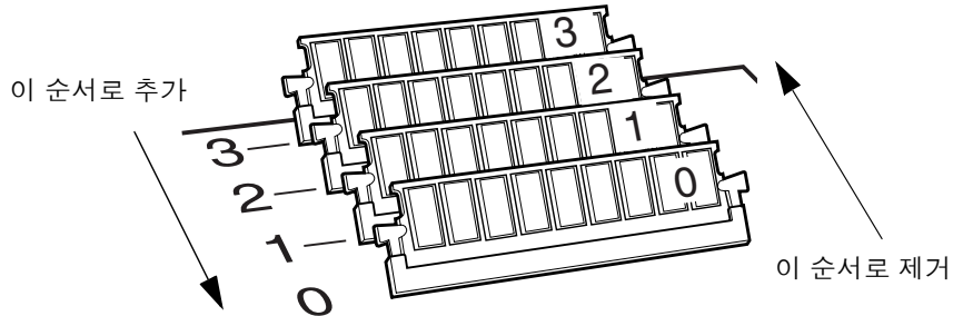
그림 8-6 DIMM 삽입 및 제거 시퀀스
