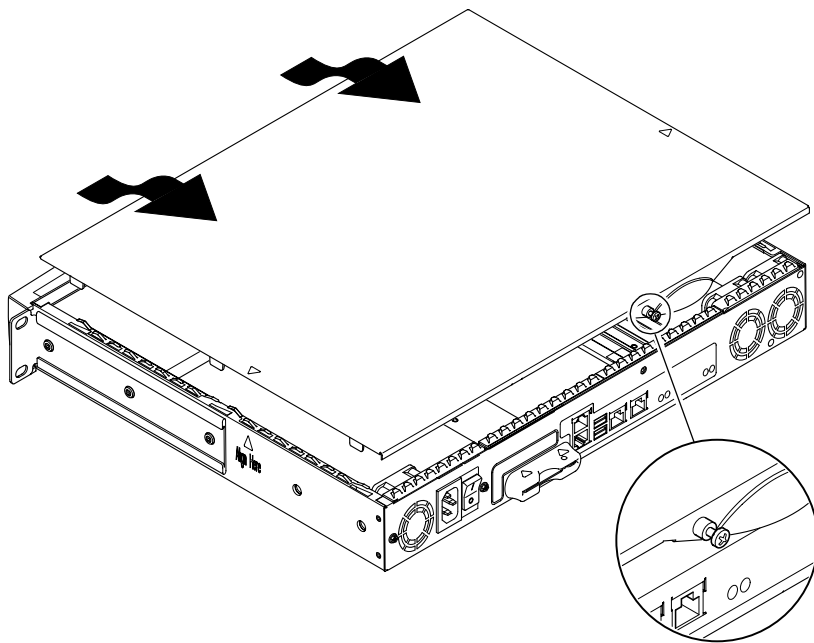
图 8-3 卸下顶盖
