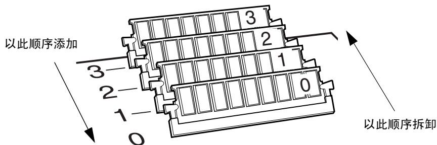
图 8-6 DIMM 插入和拆卸顺序
