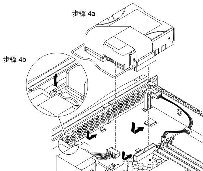
图 8-9 安装硬盘
