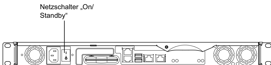
ABBILDUNG 4-1 Netzschalter „Ein/Standby“ des Netra X1 Servers
