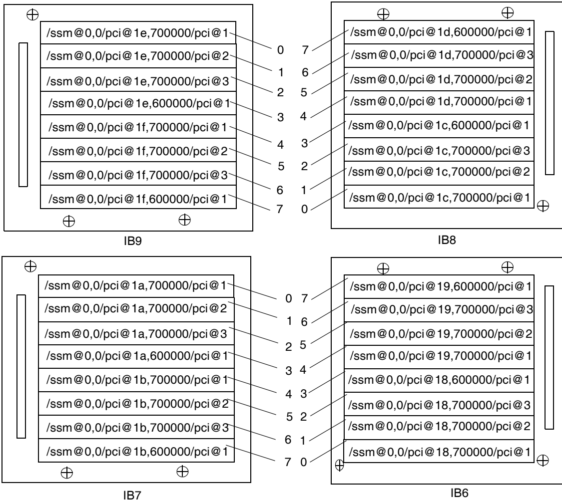
圖 A-1 IB6 至 IB9 的 Sun Fire E6900 與 6800 PCI 實體插槽指定
