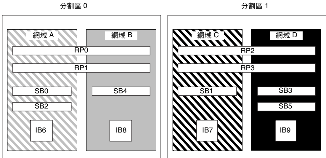
圖 1-2 雙重分割區模式下的 Sun Fire E6900 與 6800 系統
