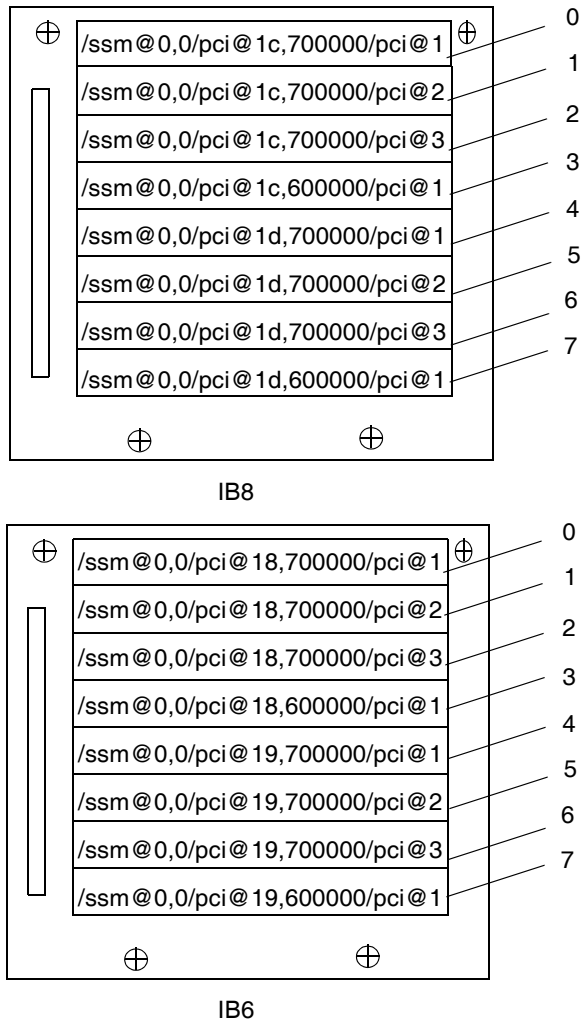
圖 A-2 IB6 與 IB8 的 Sun Fire E4900/4810/4800 系統 PCI 實體插槽指定
