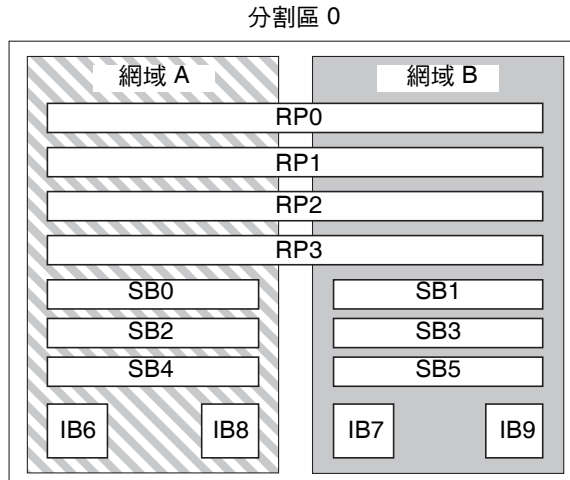
圖 1-1 單一分割區模式下的 Sun Fire E6900 與 6800 系統
