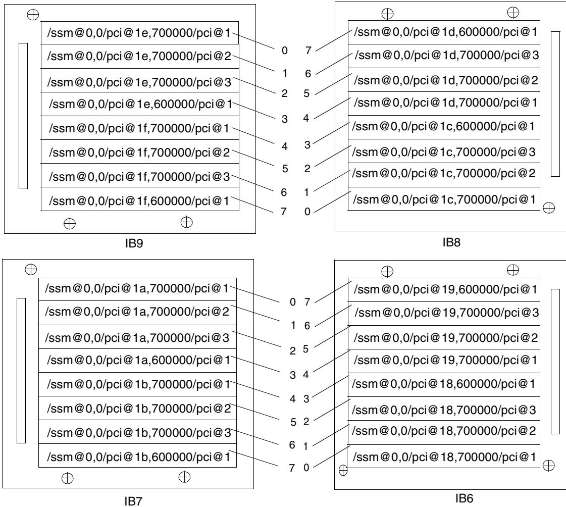
図 A-1 Sun Fire 6800 システムの IB6～IB9 に対応するシステム PCI 物理スロットの番号
