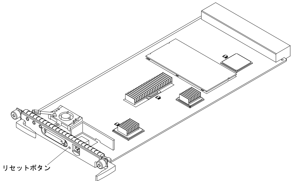
図 10-1 システムコントローラのリセット
