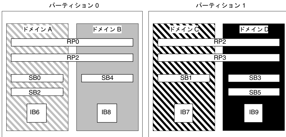
図 1-2 デュアルパーティションモードの Sun Fire 6800 システム
