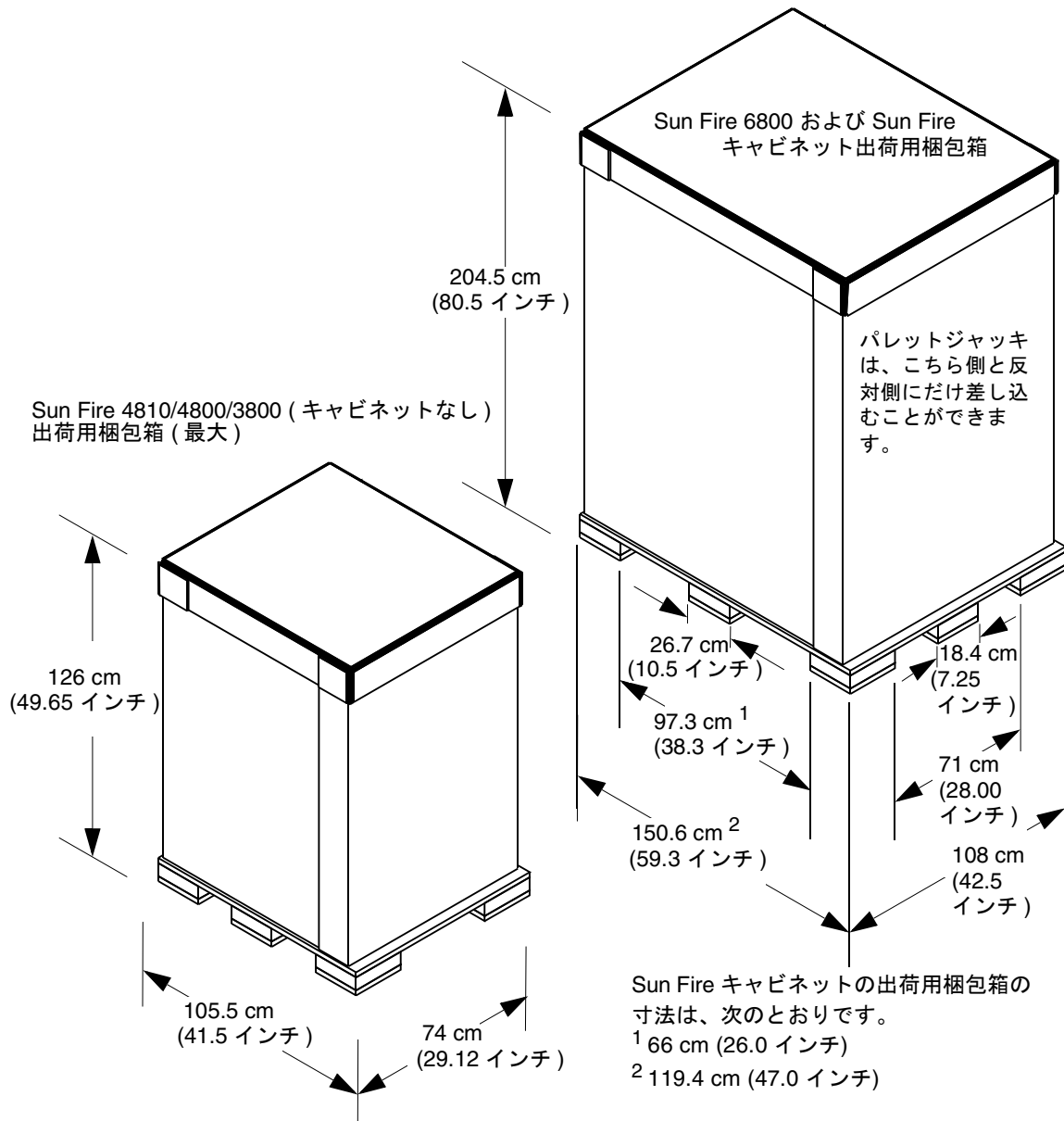
図 2-7 出荷用梱包箱の寸法
