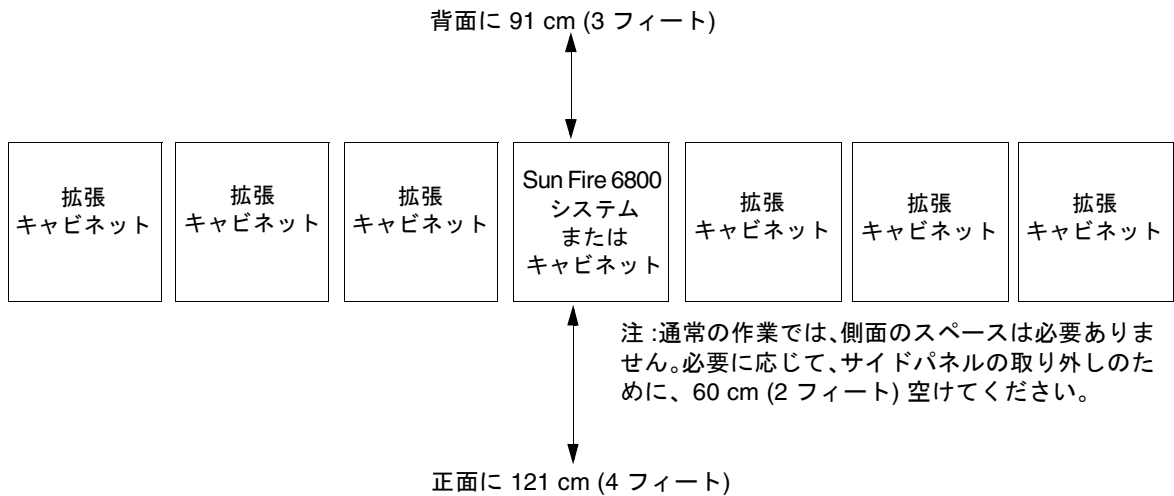
図 2-5 Sun Fire 6800/4810/4800/3800 システムのアクセス領域を上から見た図
