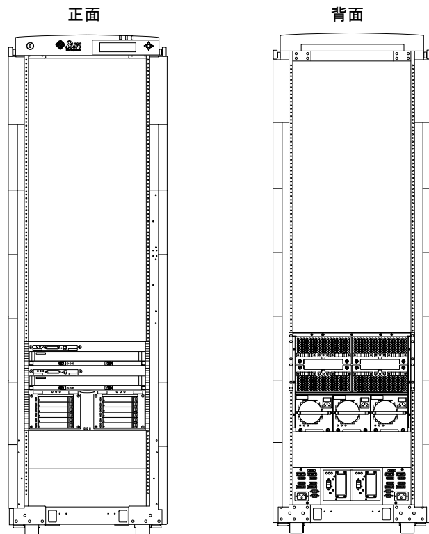
図 2-4 Sun Fire キャビネット (オプション) に搭載された Sun Fire 3800 システム
