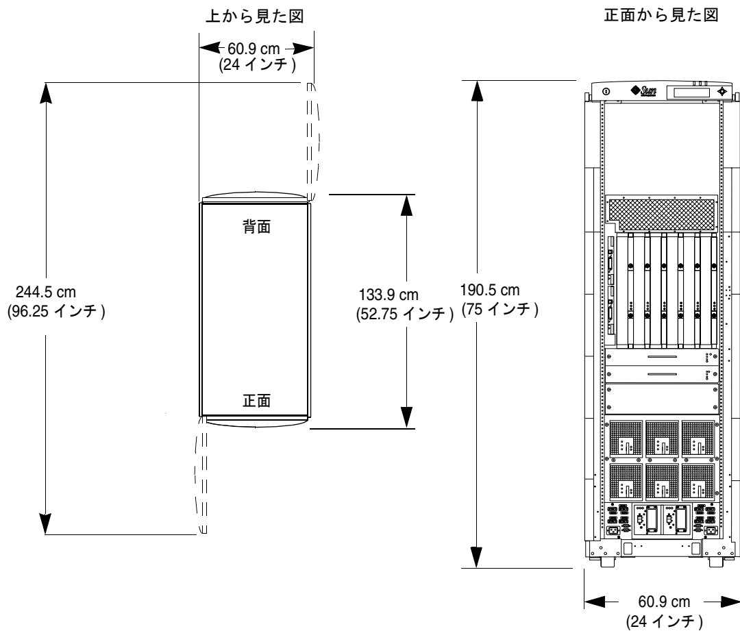
図 2-8 Sun Fire 6800 システムキャビネットの寸法
