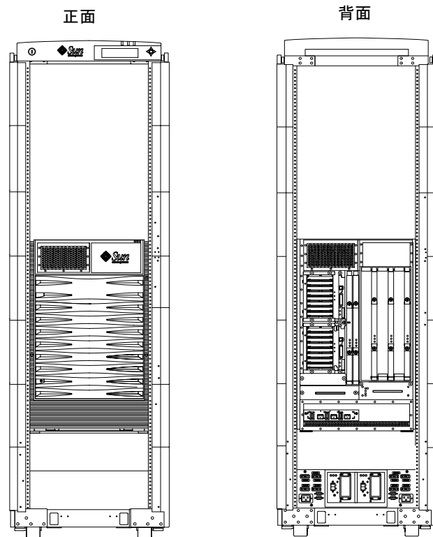
図 2-3 Sun Fire キャビネット (オプション) に搭載された Sun Fire 4800 システム
