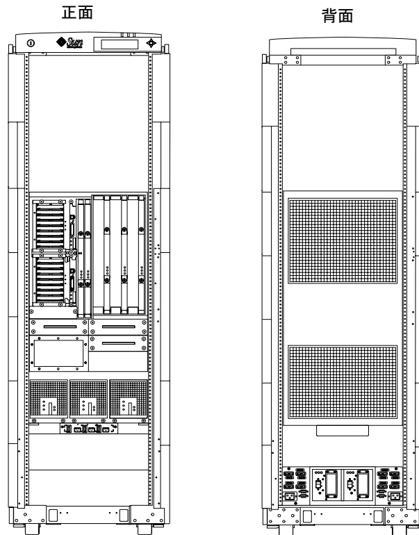
図 2-2 Sun Fire キャビネット (オプション) に搭載された Sun Fire 4810 システム
