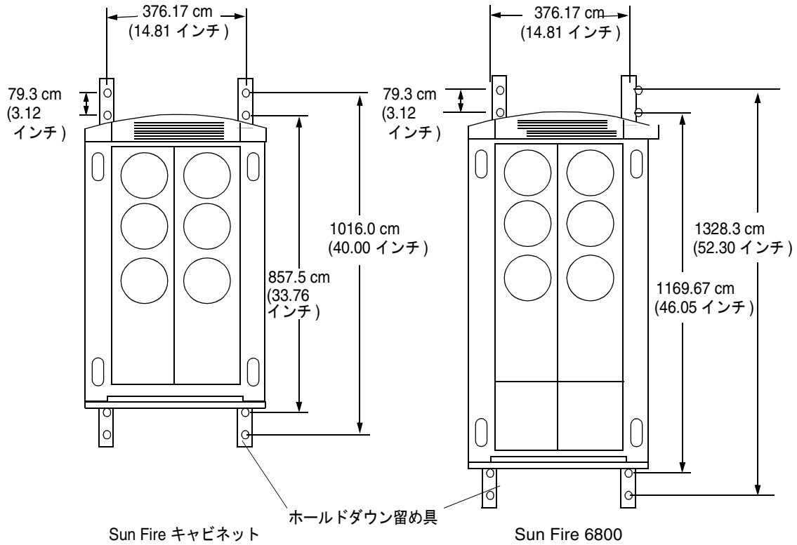
図 2-10 ホールドダウン留め具の付いた Sun Fire キャビネットおよび Sun Fire 6800 システムを上から見た図
