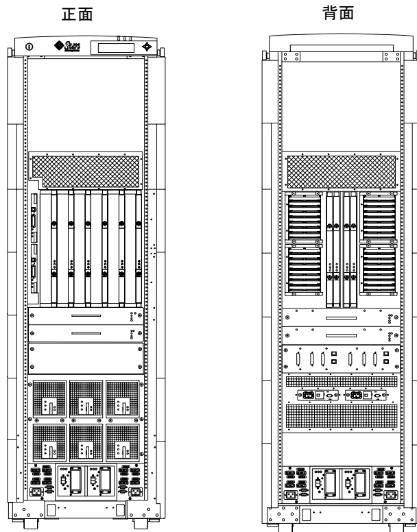
図 2-1 Sun Fire 6800 システム
