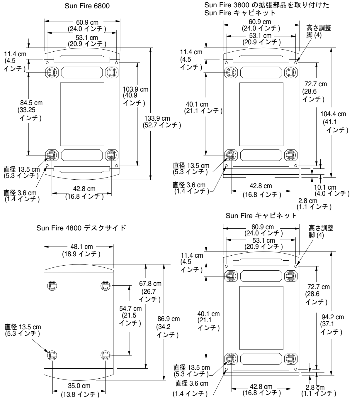
図 2-9 Sun Fire 6800/4800 および Sun Fire キャビネットを下から見た図
