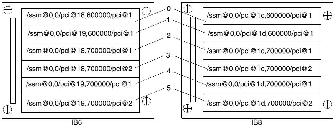
그림 A-3 Sun Fire 3800 시스템 6 슬롯 CompactPCI 물리적 슬롯 지정
