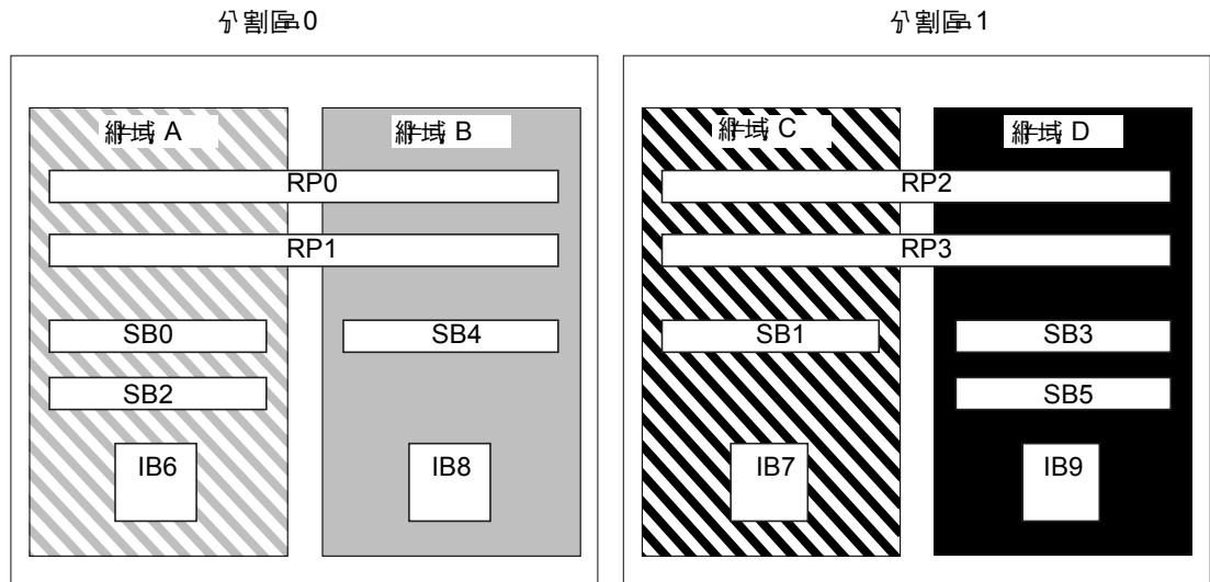
圖 1-2 雙重分割區模式下的 Sun Fire E6900 和 6800 系統
