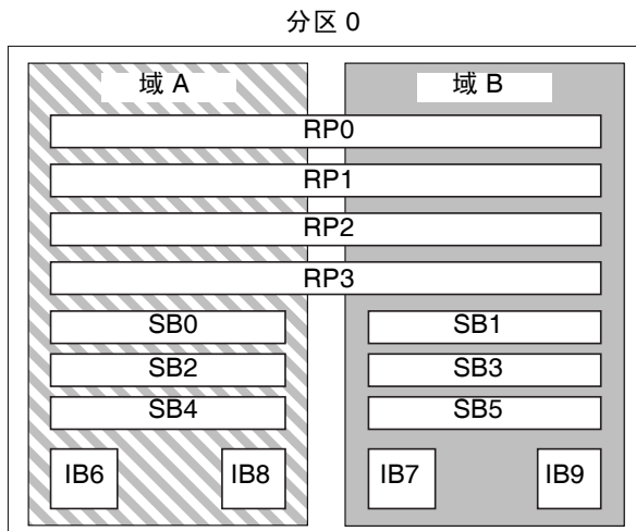
图 1-1 Sun Fire E6900 和 6800 系统（单分区模式）
