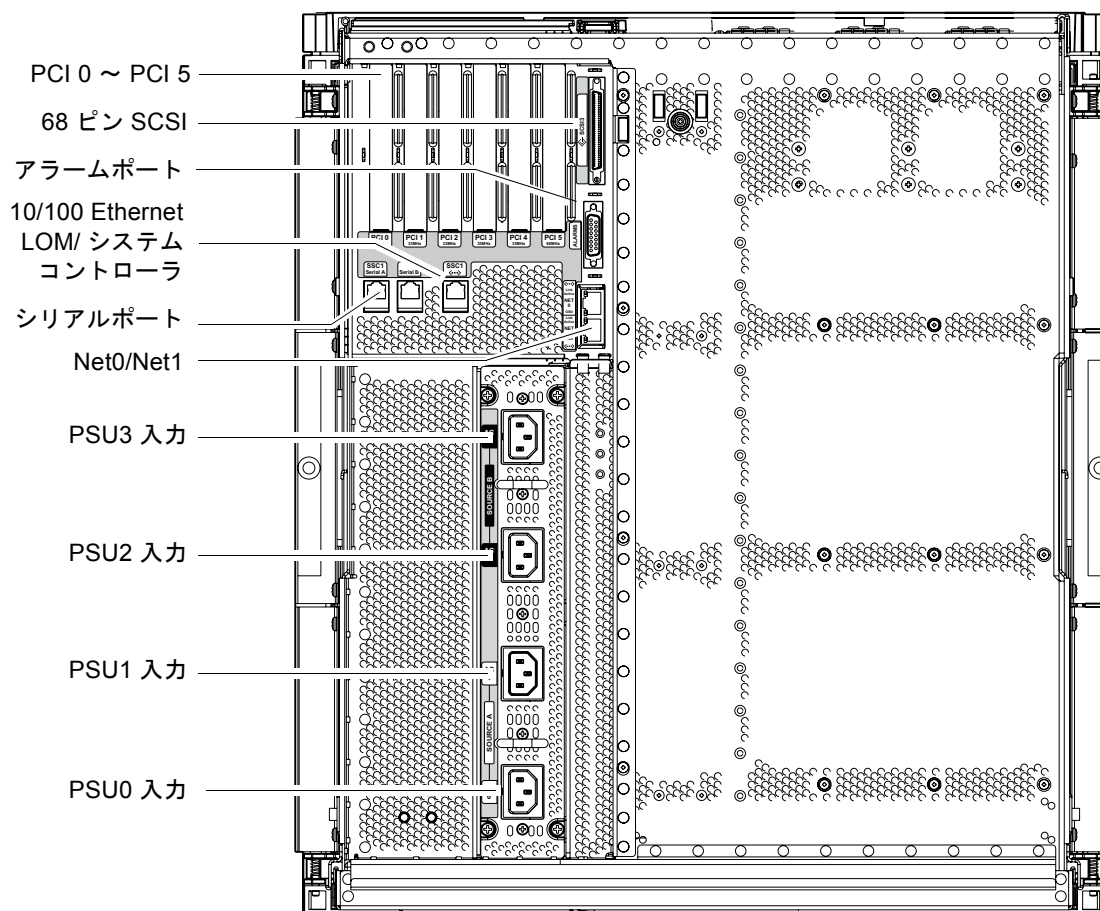
図 1-1 I/O ポート
