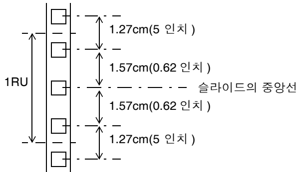
그림 2-1 EIA/RETMA 범용 마운팅 구멍 패턴 치수
