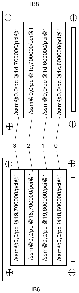
그림 A-4 Sun Fire E4900/4810/4800 시스템에서 4 슬롯 CompactPCI 물리적 슬롯 지정
