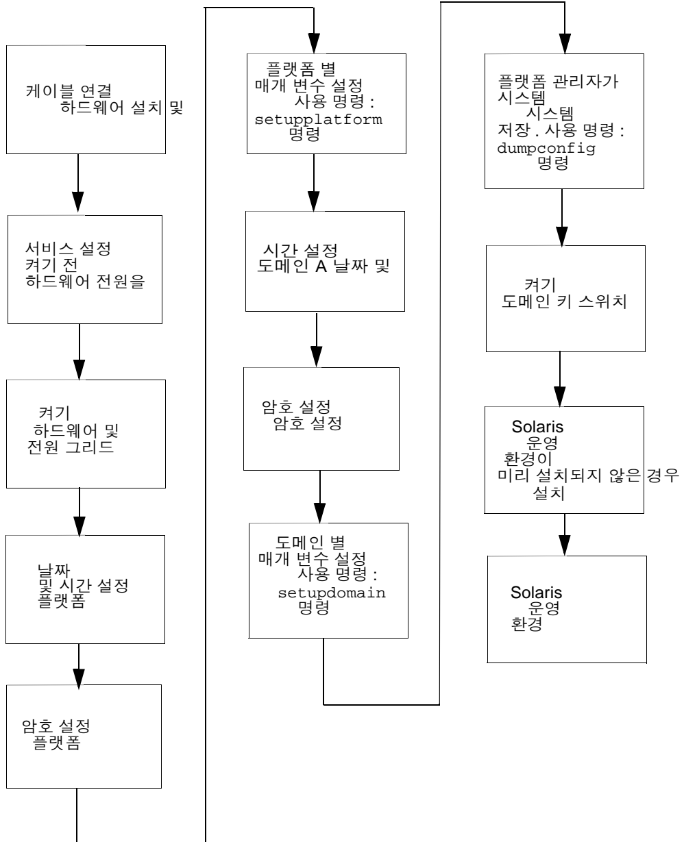
그림 3-1 시스템 전원 켜기 및 설정 단계 플로우차트
