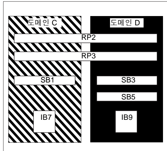
그림 1-2 이중 분할 영역 모드의 Sun Fire E6900 및 6800 시스템
