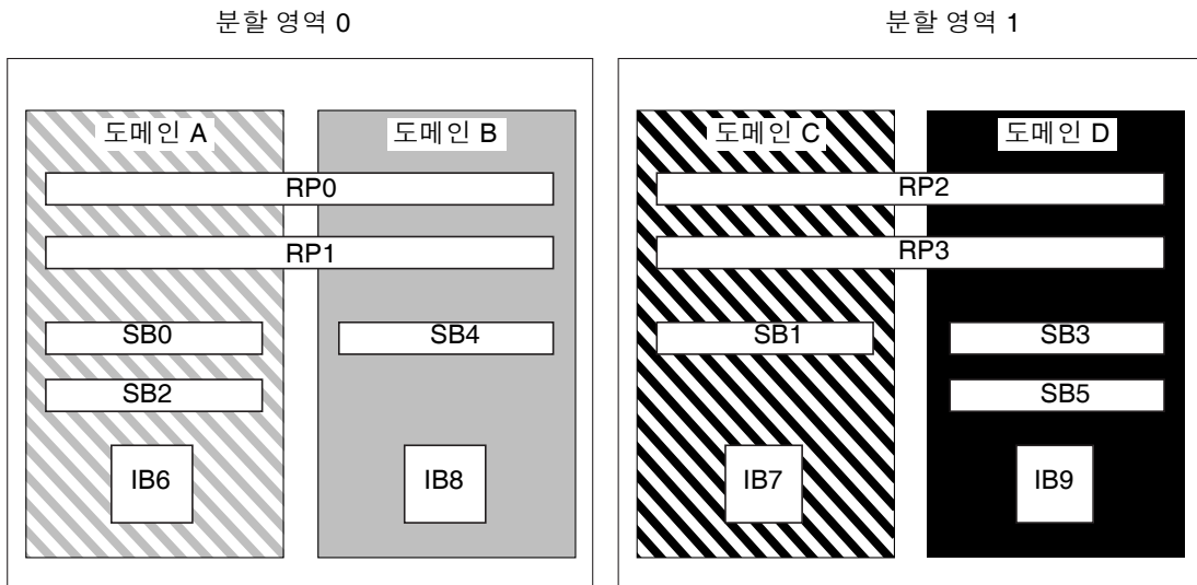
그림 1-2 이중 분할 영역 모드의 Sun Fire E6900 및 6800 시스템
