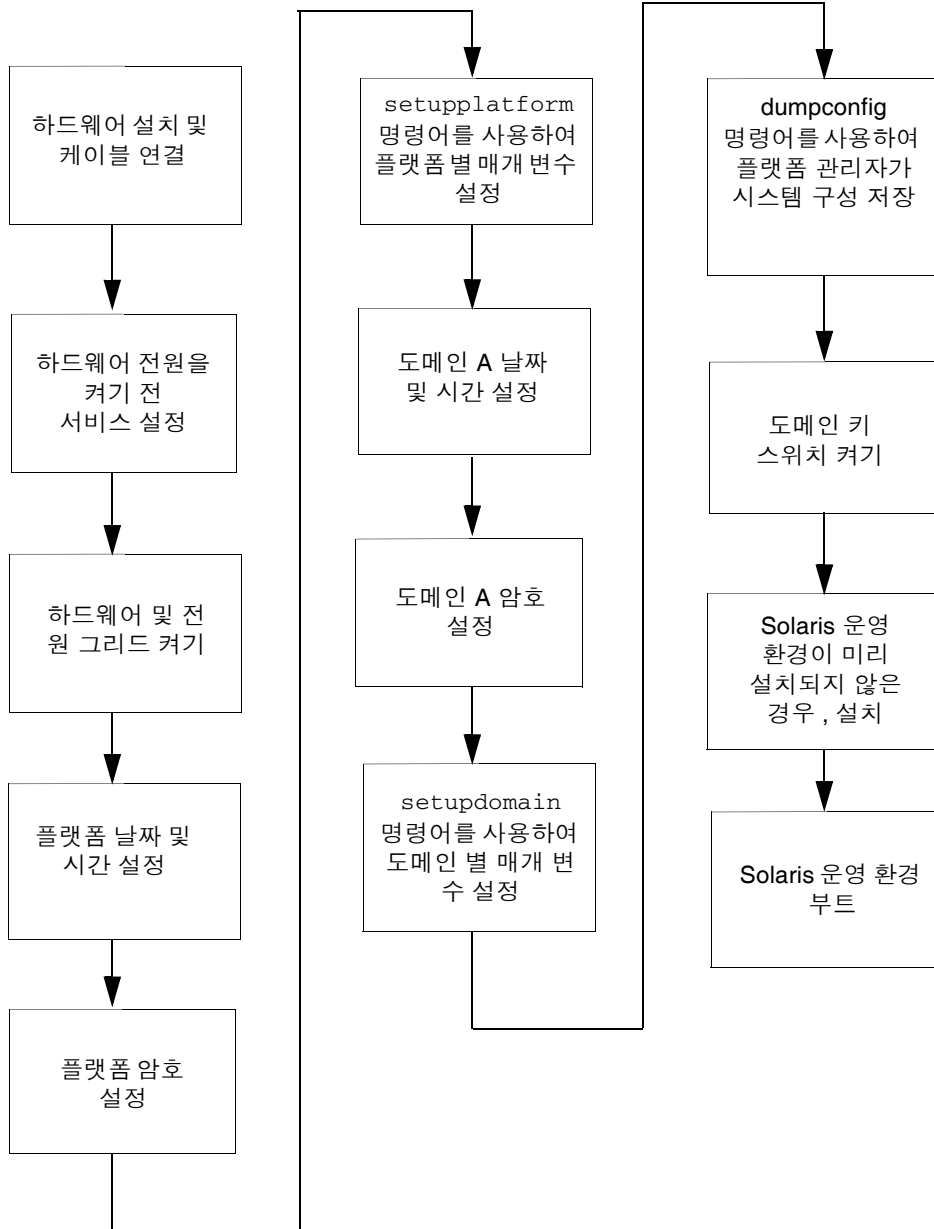
그림 3-1 시스템 전원 켜기 및 설정 단계 플로우차트
