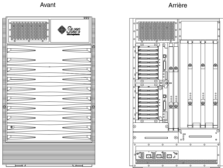
FIGURE 1-3 Système Sun Fire E4900 - Vues avant et arrière
