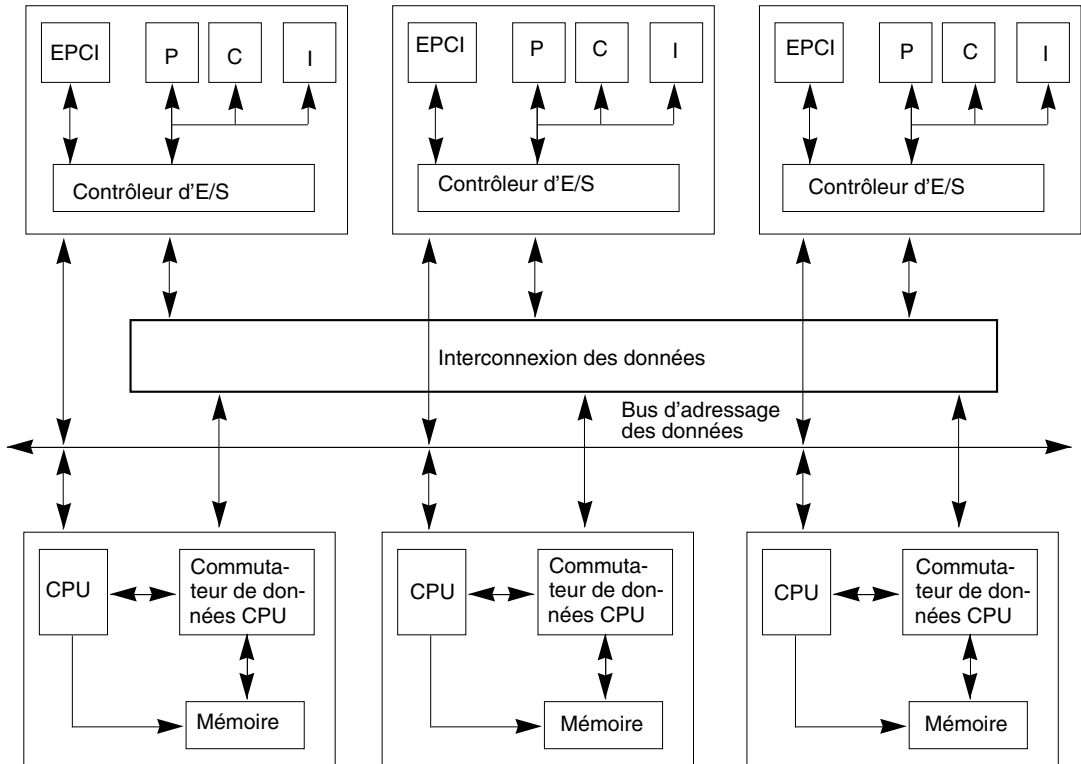
FIGURE 3-1 Fonctionnement standard des systèmes Sun Fire E6900/E4900
