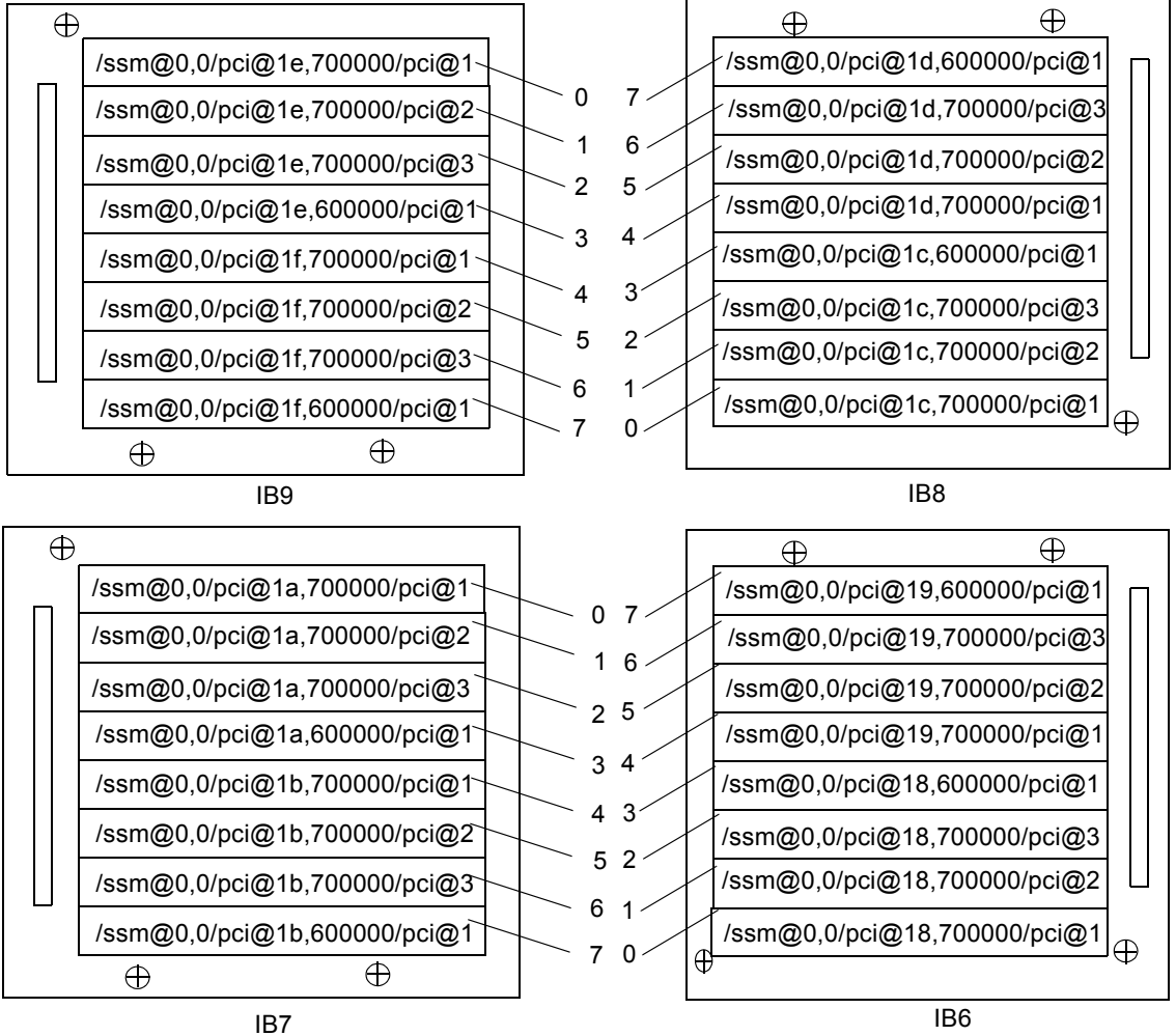
그림 A-1 Sun Fire E6900 및 6800에서 IB6에서 IB9까지의 PCI 물리적 슬롯 지정
