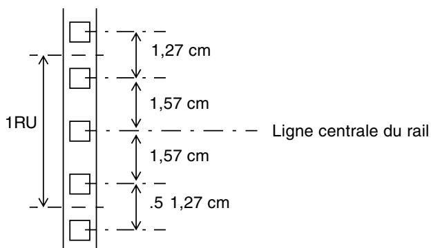
FIGURE 2-1 Espacement des trous de montage EIA/RETMA
