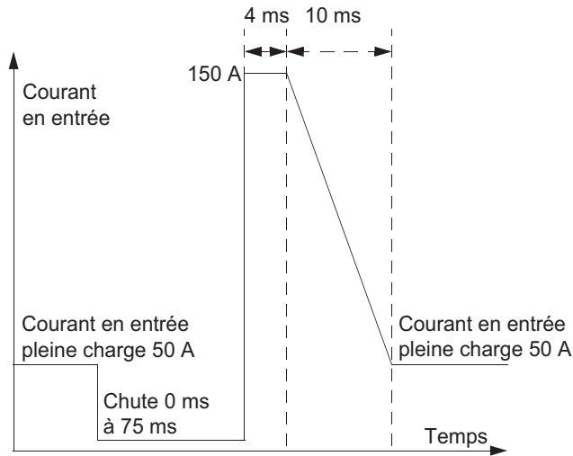
FIGURE 3-1 Courant de choc
