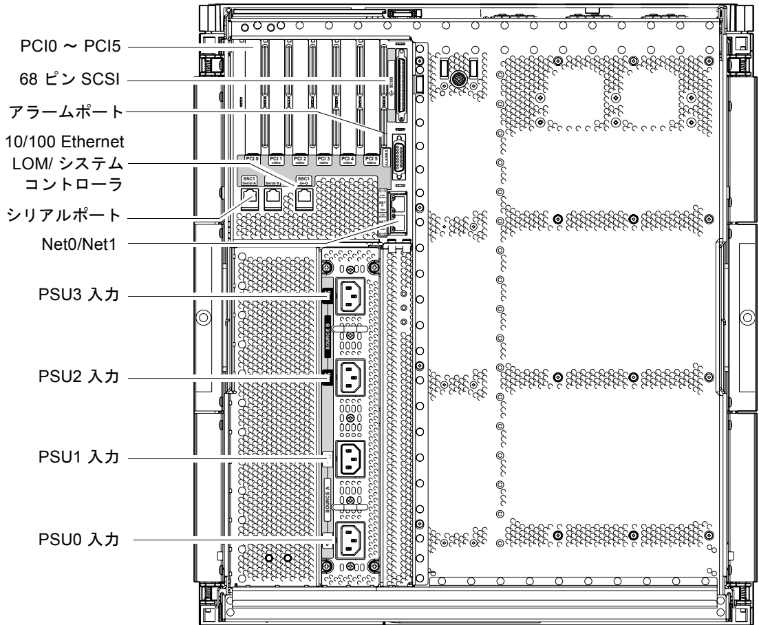
図 1-1 I/O ポート
