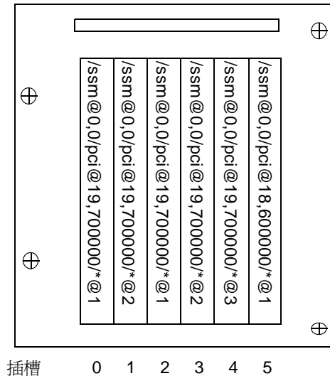
圖 10-1 IB6 的 Sun Fire 入門級中階系統 IB_SSC PCI 實體插槽指定
