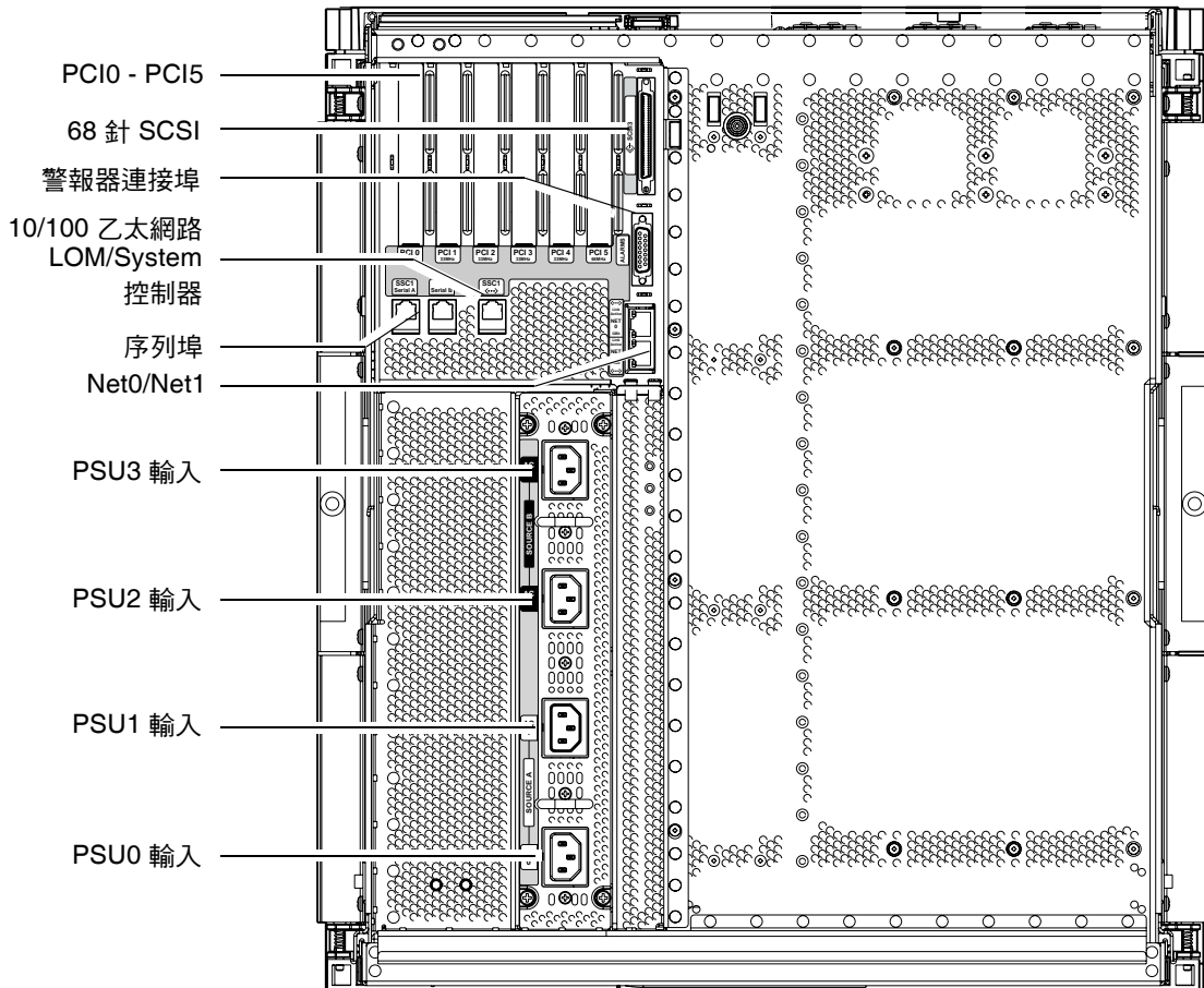
圖 1-1 I/O 連接埠
