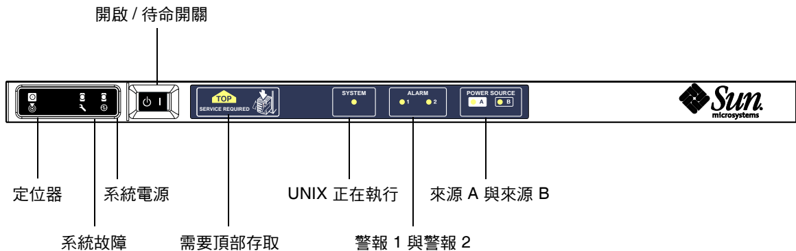
圖 10-2 系統指示燈
