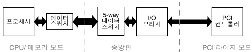
그림 6-3 여러 FRU를 통해 실행되는 POST 진단
