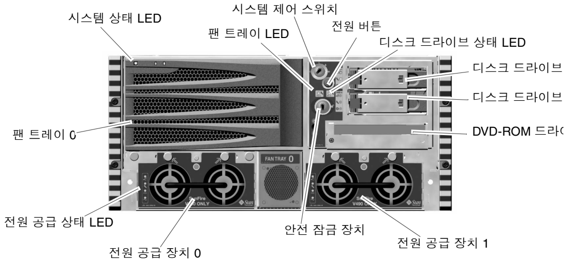
그림 2-1 Sun Fire V490 서버 전면 패널 기능
