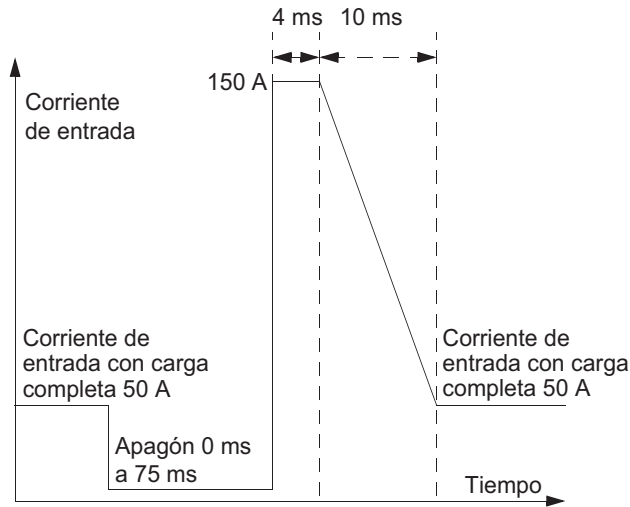
FIGURA 3-1 Sobrecorriente momentánea
