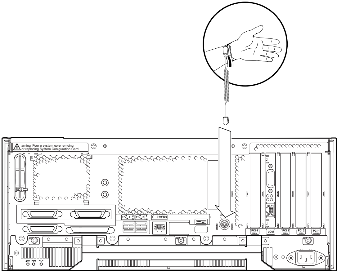
그림 12-1 새시의 후면에 정전기 방지 손목 띠 부착
