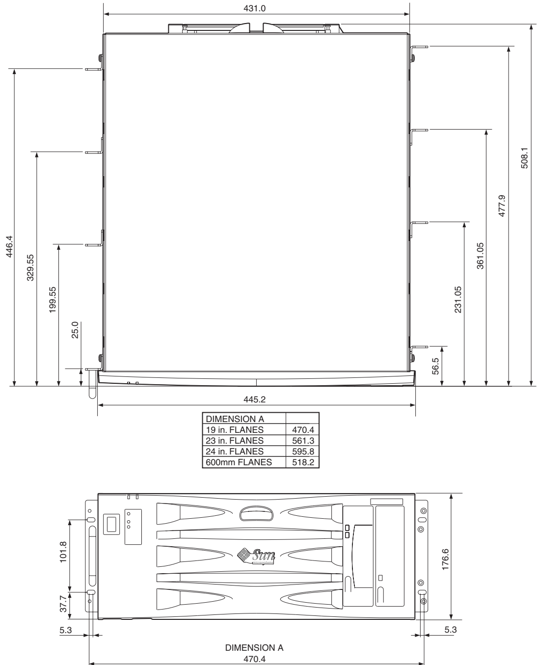
그림 2-1 Netra T4 시스템 크기 및 설치 옵션(크기는 mm)
