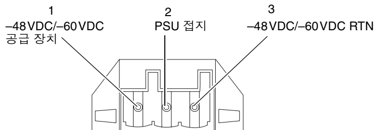
그림 3-6 DC 전원 공급 장치의 전원 커넥터
