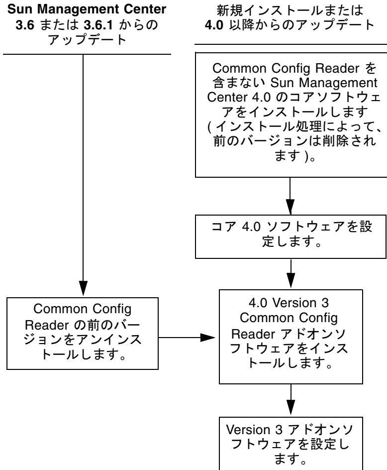
図 1 インストール処理の流れ
