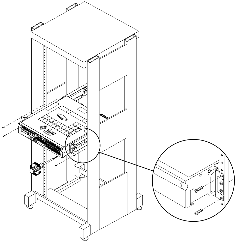
FIGURA 3-22 Fijación de la parte frontal del servidor al frontal del bastidor
