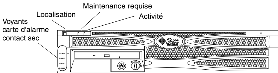
FIGURE 1-2 Emplacement des indicateurs du panneau avant
