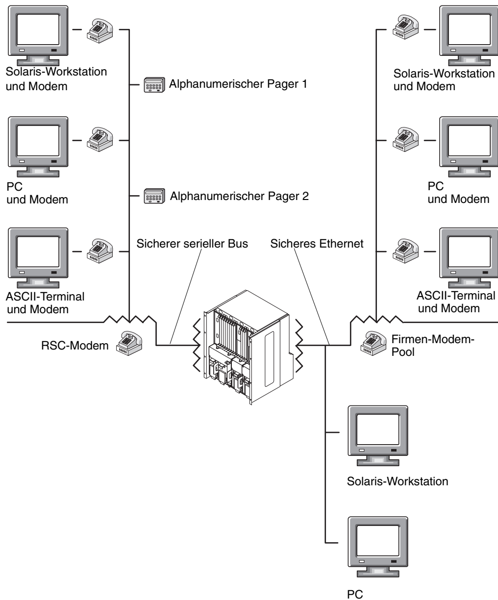
ABBILDUNG 1-2 Möglichkeiten für die RSC-Fernbenachrichtigung
