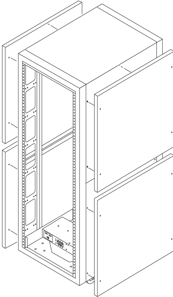
그림 4-1 측면 패널 제거 및 다시 끼우기
