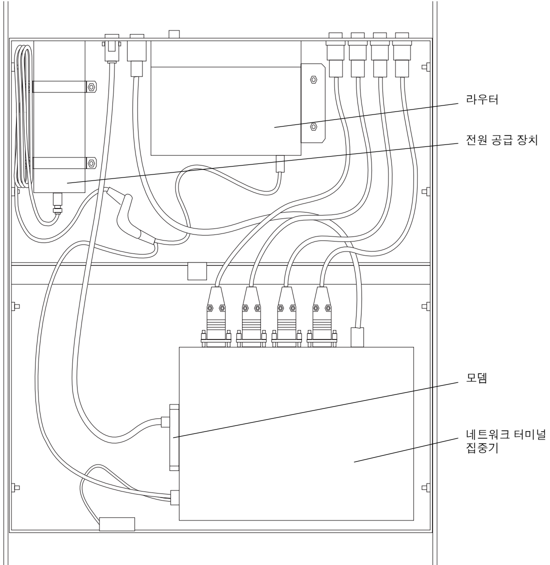
그림 4-18 Storage Service Processor 액세스러리 트레이의 내부 구조
