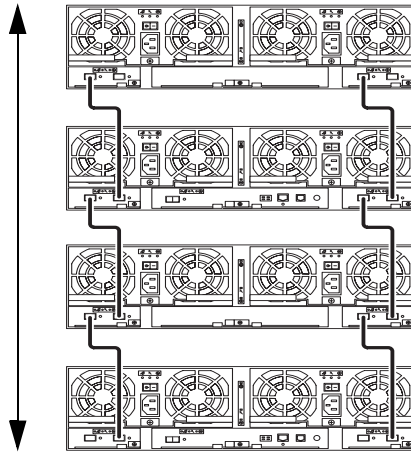
그림 4-15 2×4 HA 구성 및 해당 트레이 번호
