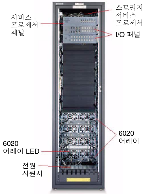
그림 1-2 Sun StorEdge 6320 시스템 - 후면
