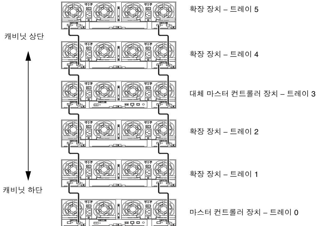
그림 4-16 2x6 HA 구성 및 해당 트레이 번호
