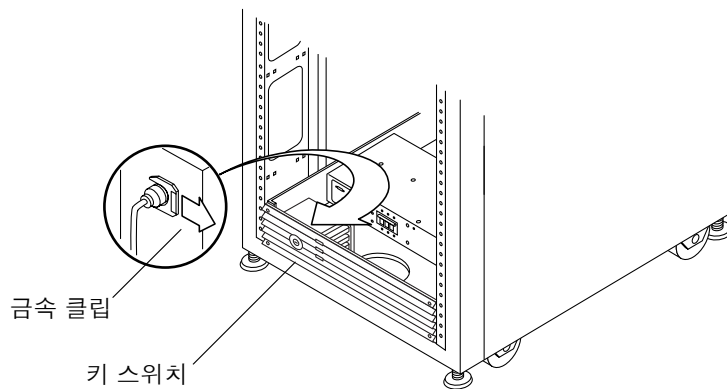
그림 4-10 키 스위치 제거 및 재설치
