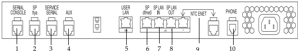
그림 4-17 Storage Service Processor 액세스리 트레이 연결부
