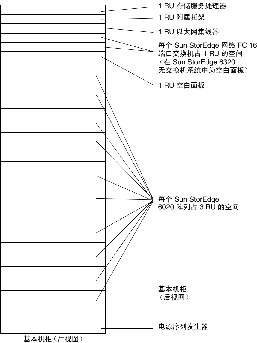
图 4-3 Sun StorEdge 6320 系统 FRU 布置
