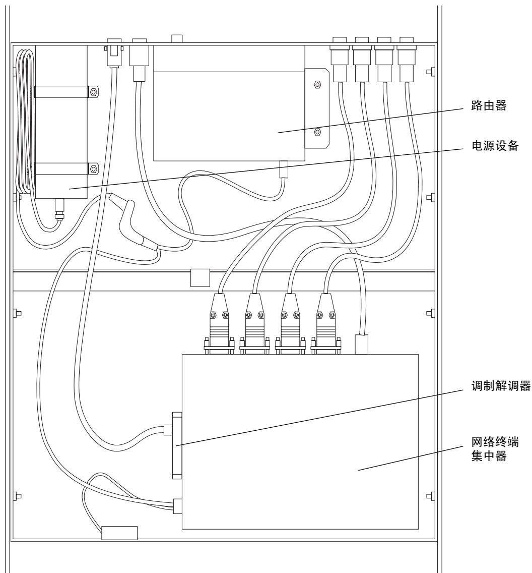
图 4-18 存储服务处理器附属托架的内部布局
