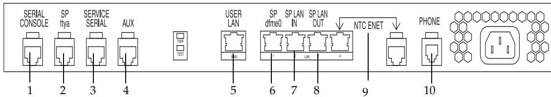
图 4-17 存储服务处理器附属托架接口
