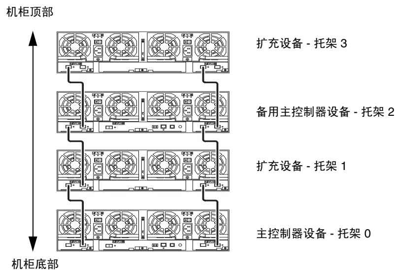
图 4-15 2x4 HA 配置和相应的托架编号
