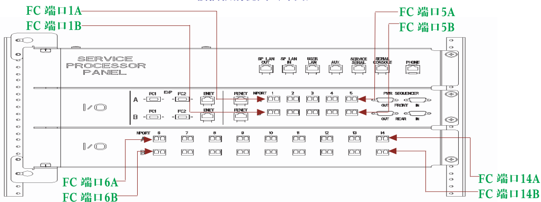
接插板后视图（内侧）
