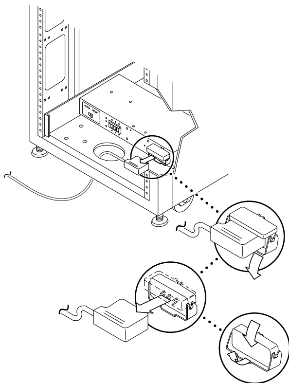
图 4-8 拔下交流电源线插头
