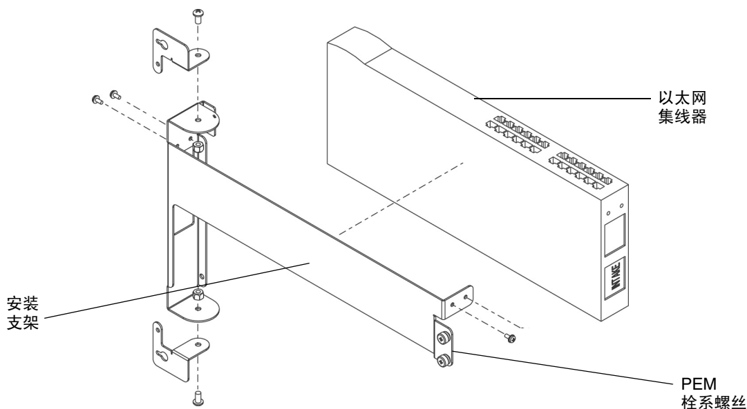
图 4-11 从第二个机柜中拆卸以太网集线器
