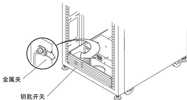
图 4-10 拆卸和装回钥匙开关
