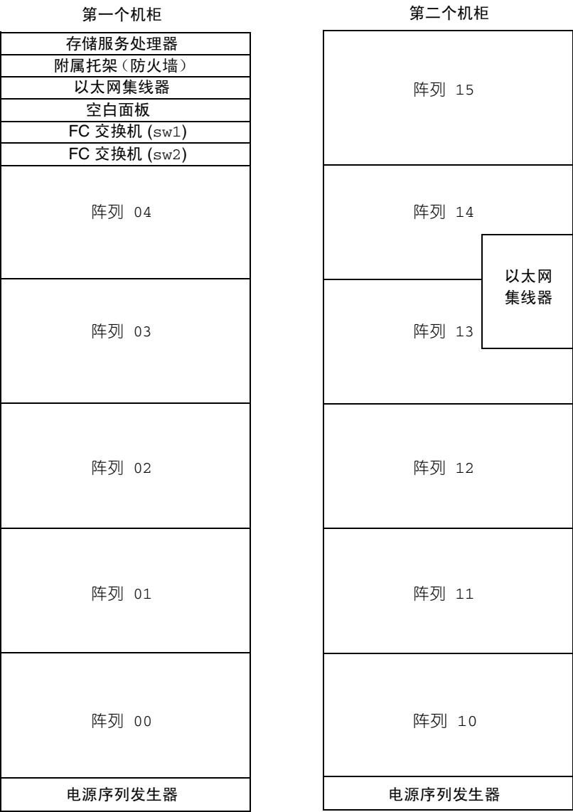
图 1-5 Sun StorEdge 6320 系统的后视图
