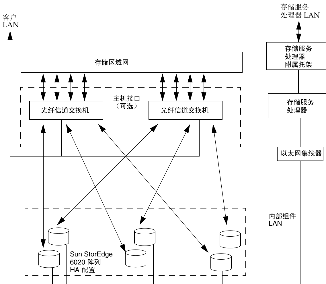
图 1-4 基本 Sun StorEdge 6320 系统体系结构
