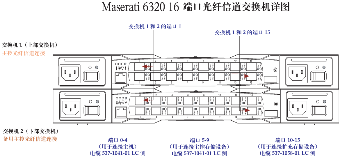
图 C-2 16 端口光纤信道交换机详图
