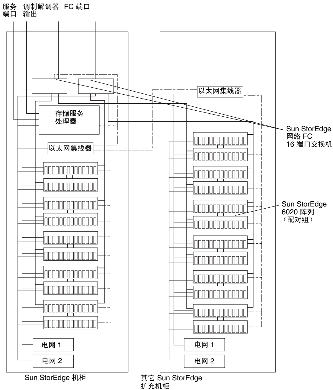
图 1-3 Sun StorEdge 6320 系统
