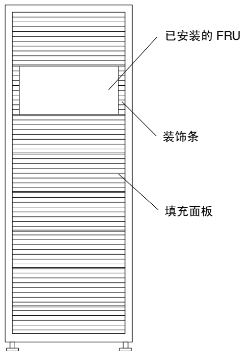
图 4-5 填充面板和装饰条位置
