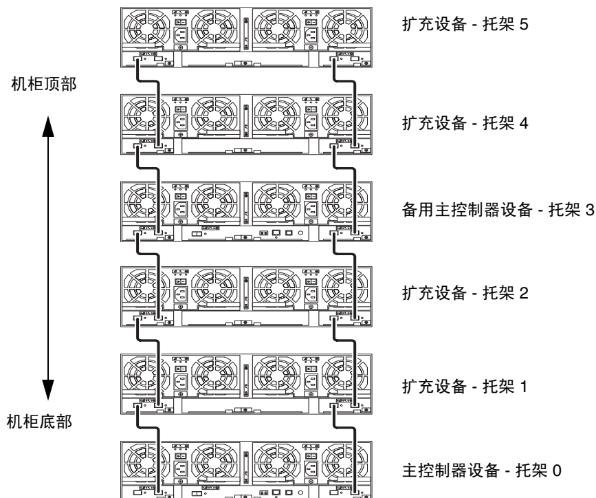
图 4-16 2×6 HA 配置和相应的托架编号
