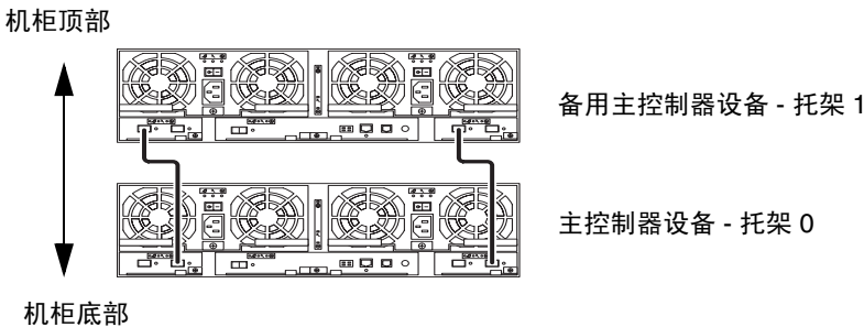
图 4-14 2x2 HA 配置和相应的托架编号
