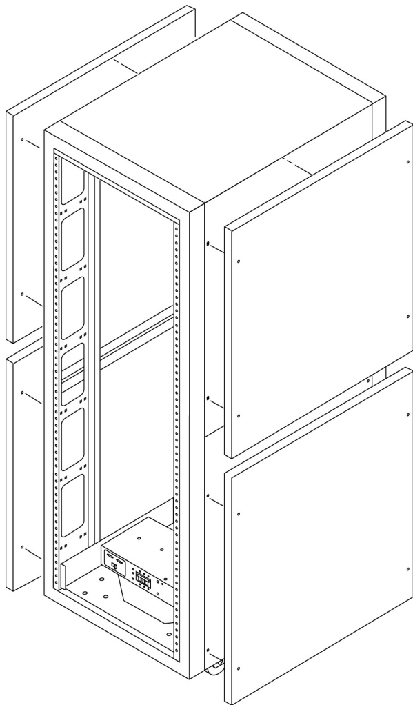
图 4-1 拆卸和装回侧面板
