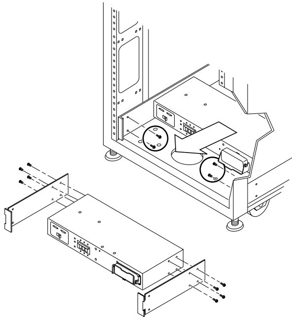
图 4-7 拆卸电源序列发生器
