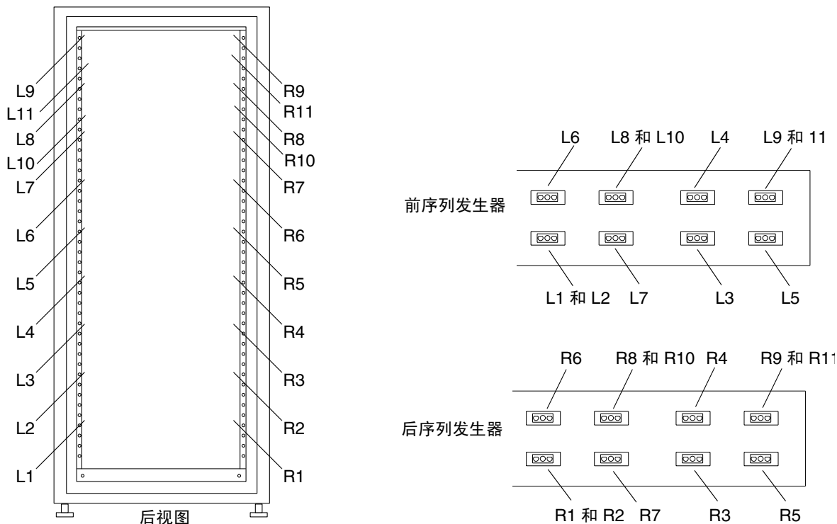
图 4-6 电源线连接
