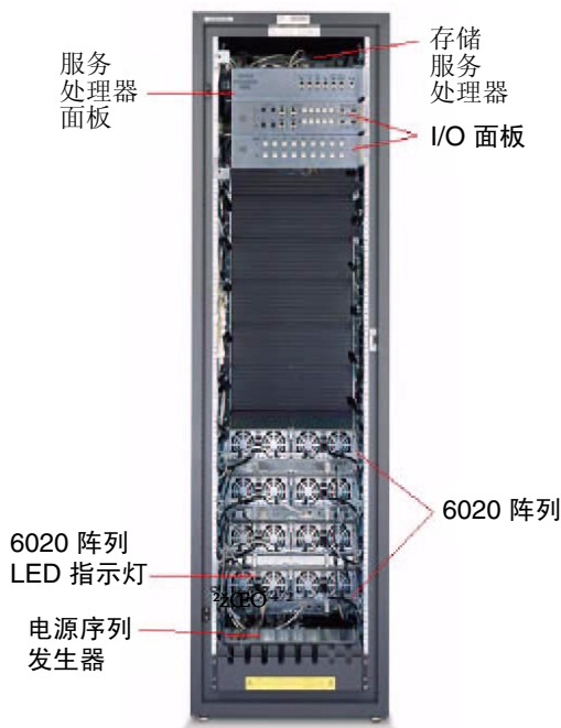
图 1-2 Sun StorEdge 6320 系统 - 后视图
