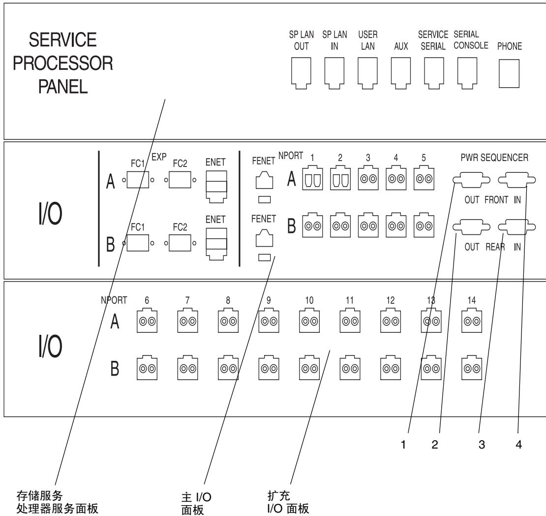
图 4-12 存储服务处理器服务面板上连接器的前视图
