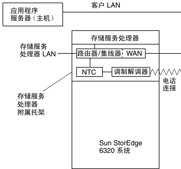
图 1-7 具有远程服务的单个 Sun StorEdge 6320 系统
