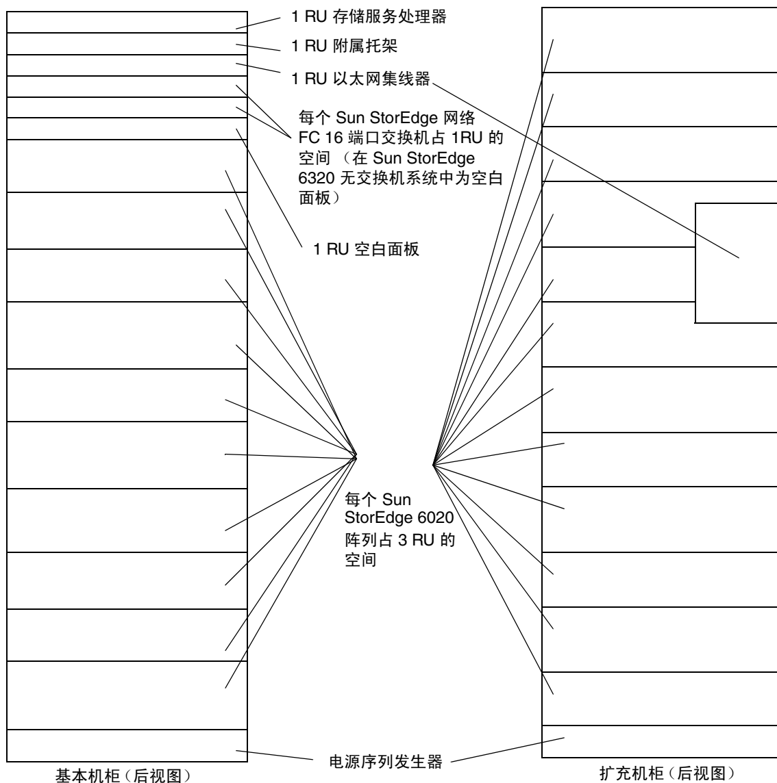
图 4-4 Sun StorEdge 6320 系统 FRU 位置
