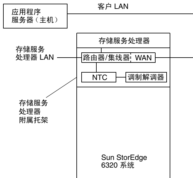
图 1-6 没有远程服务的单机 Sun StorEdge 6320 系统
