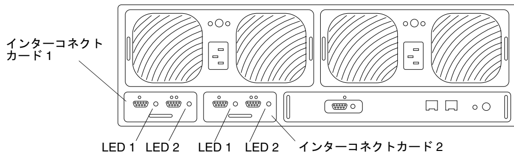
図 5-6 Sun StorEdge T3 ディスクトレイ背面パネル上のインターコネクトカード
