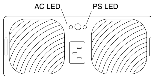
図 5-2 Sun StorEdge T3 ディスクトレイ背面パネルにある電源・冷却装置
