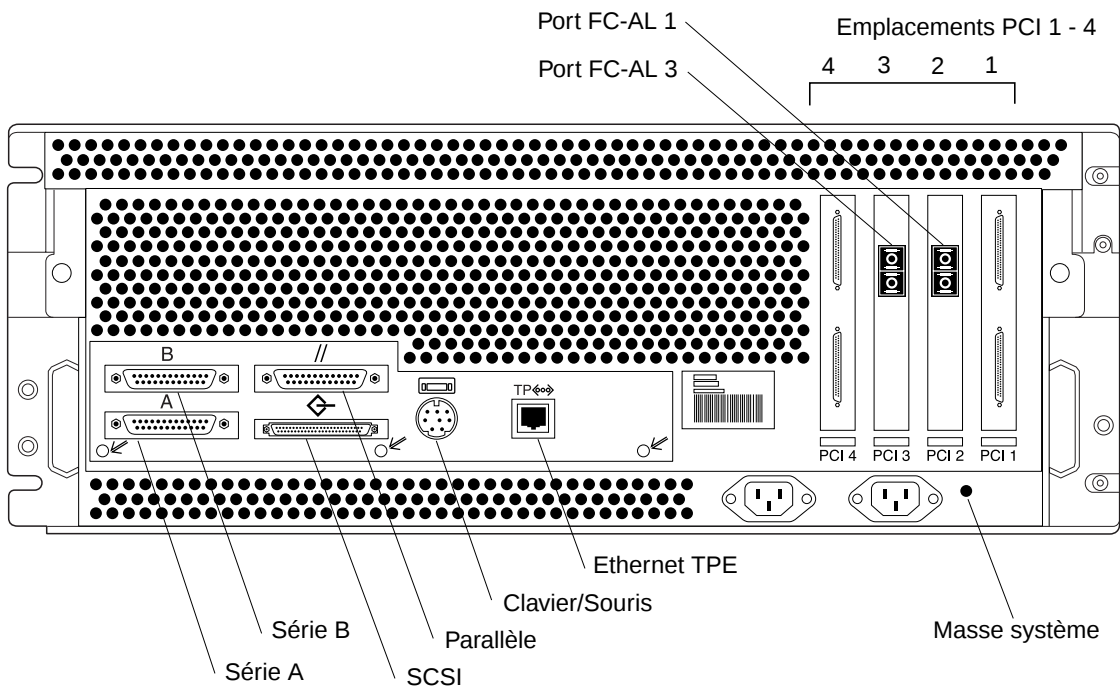
FIGURE 8 Détails et connexions du panneau arrière du serveur Sun Enterprise 420R
