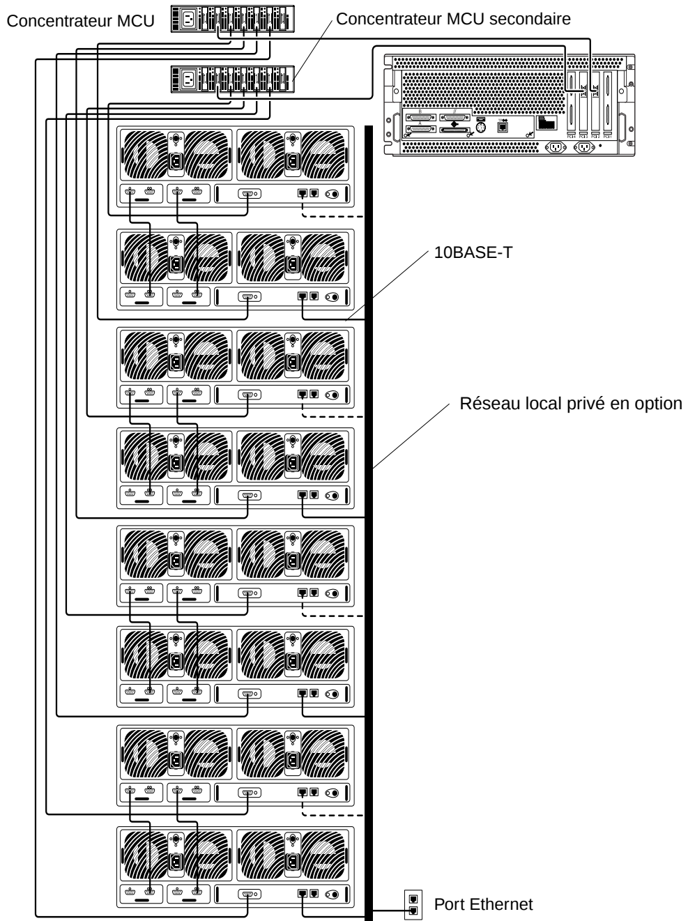
FIGURE 9 Configuration maximale pour Sun StorEdge N8400 Filer
