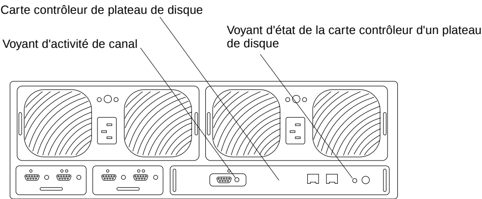
FIGURE 12 Arrière du plateau de disque Sun StorEdge T3
