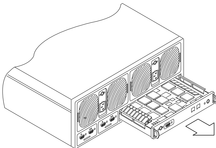
FIGURE 13 Retrait de la carte contrôleur de SunStorEdge T3
