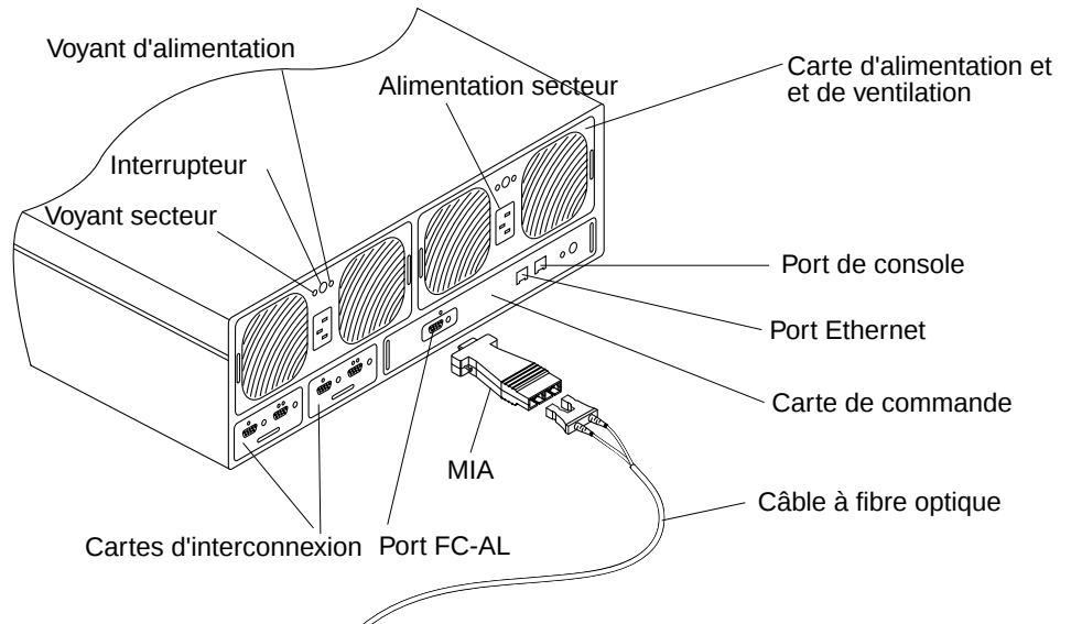
FIGURE 6 Détails du panneau arrière d'un plateau de disque
