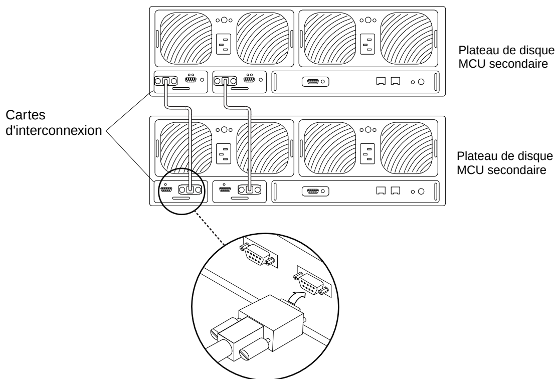
FIGURE 5 Branchement des câbles d'interconnexion
