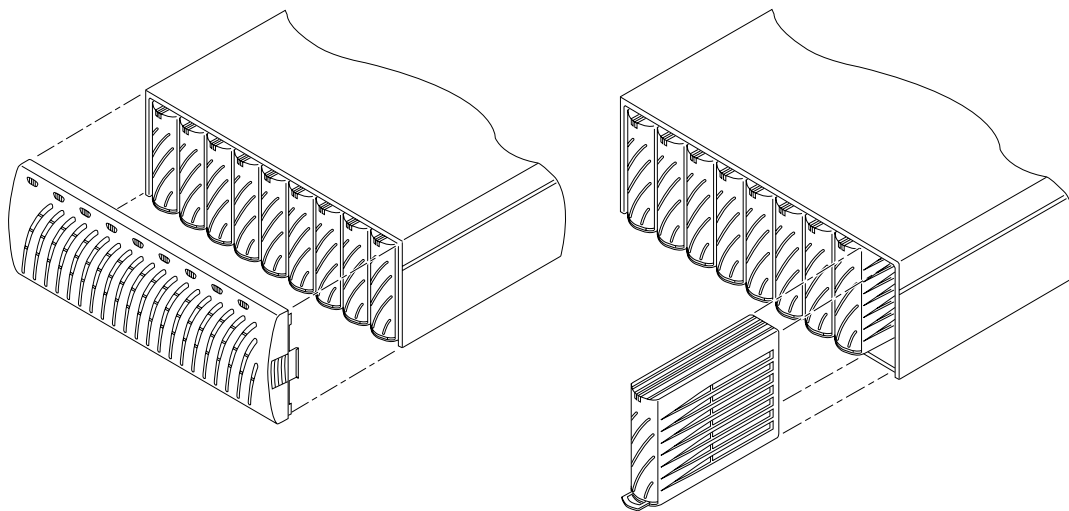
FIGURE 11 Retrait du panneau avant et d'une unité de disque d'un plateau de disque
