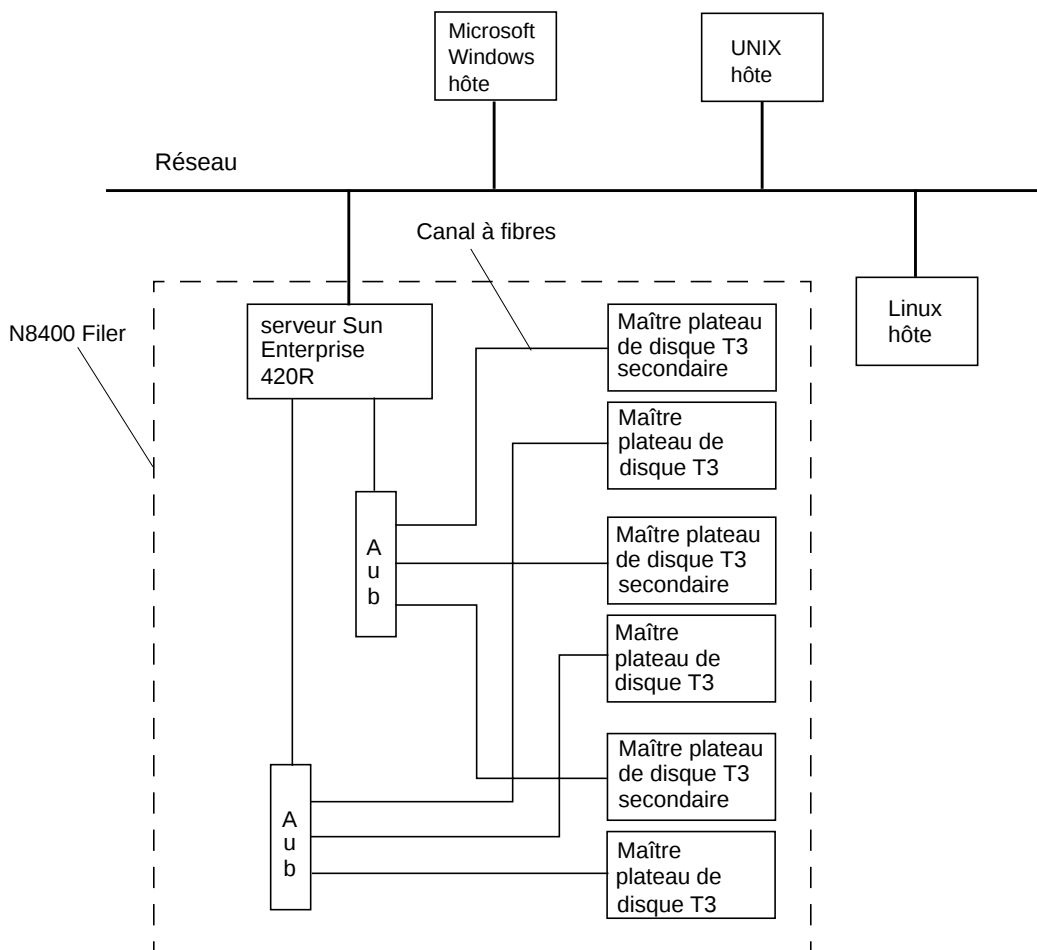
FIGURE 2 Exemple de système Sun StorEdge N8400 Filer
