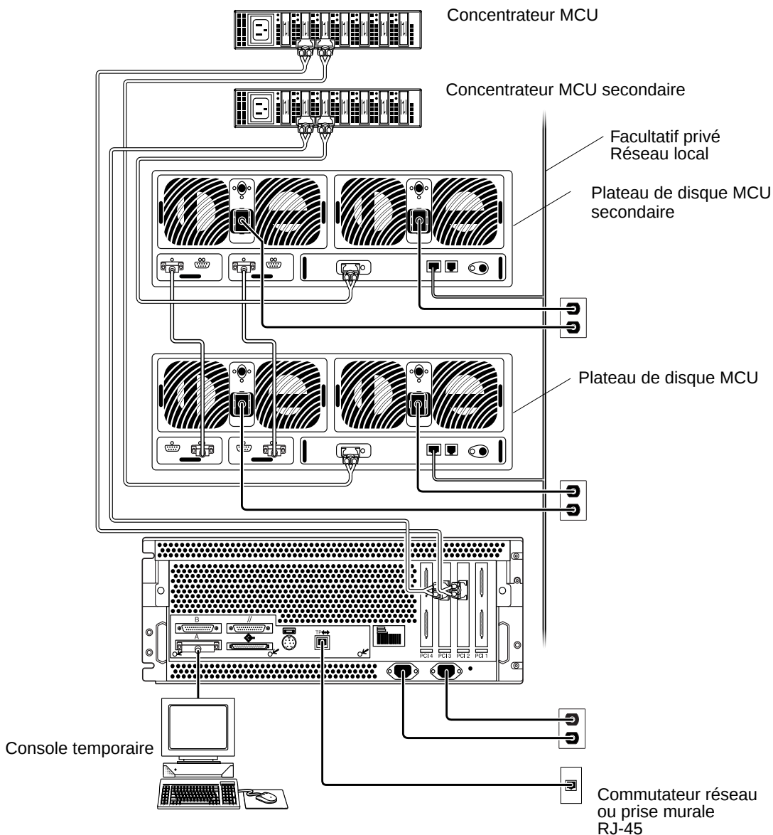
FIGURE 7 Connexions entre le serveur Sun Enterprise 420R et un groupe partenaire de plateaux de disque à des fins d'installation
