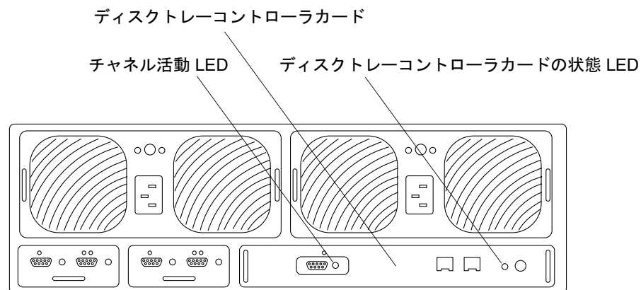
図 12 Sun StorEdge T3 ディストレーの背面
