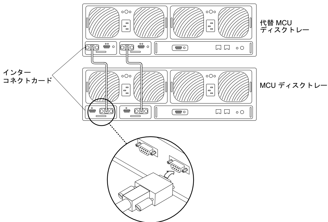
図 5 インターコネクトケーブルの接続
