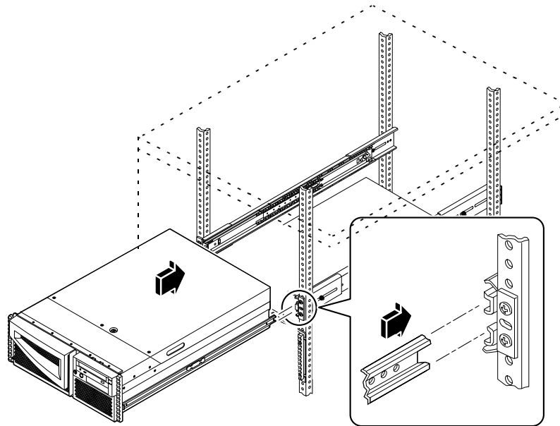
図 4 Sun Enterprise 420R Server の設置
