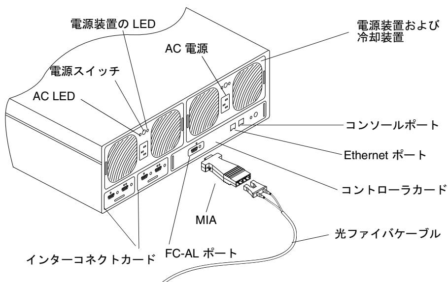
図 6 ディスクトレイの背面パネルの詳細
