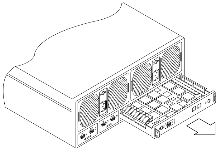
図 13 SunStorEdge T3 コントローラカードの取り外し
