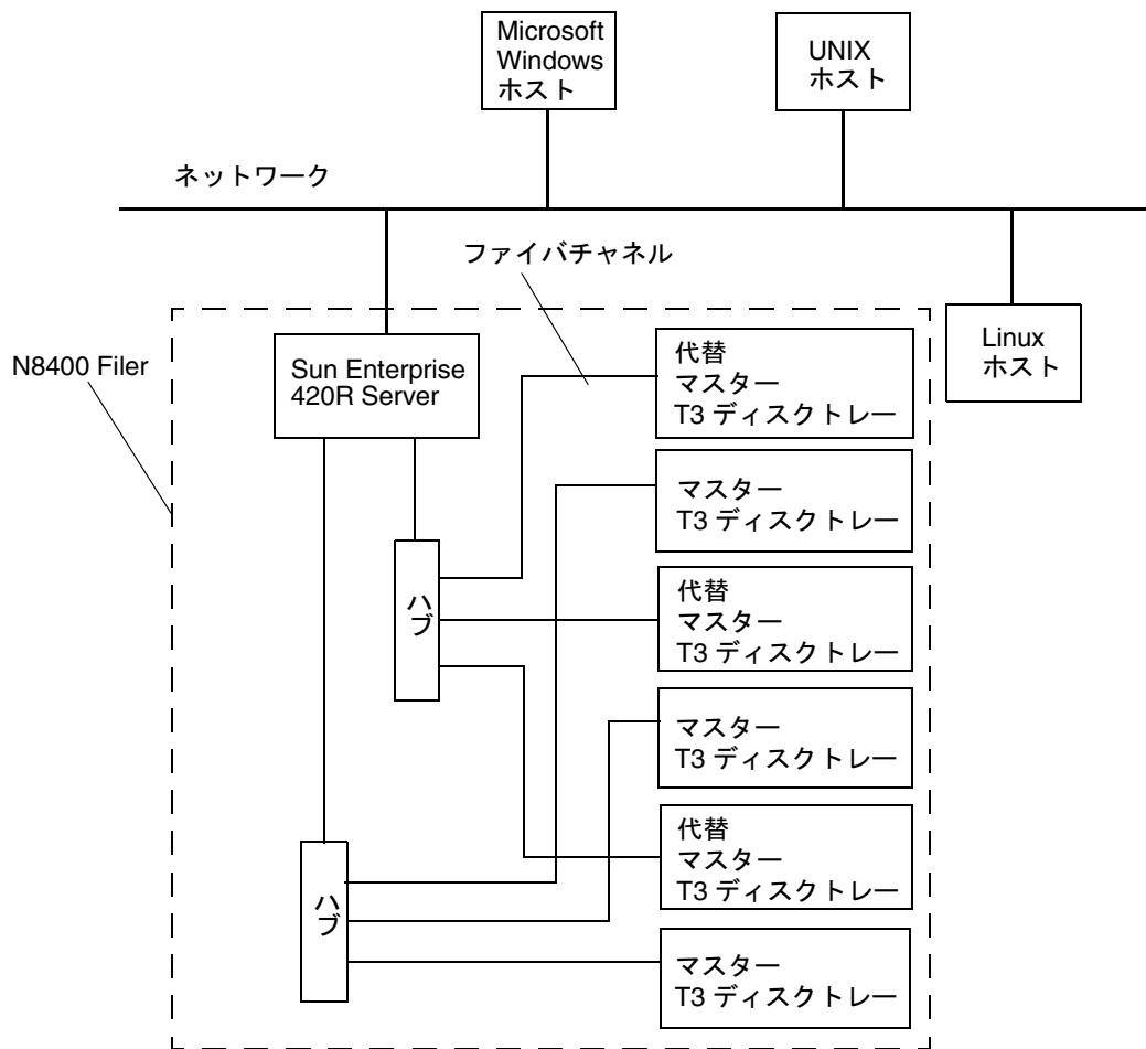
図 2 Sun StorEdge N8400 Filer システムの例
