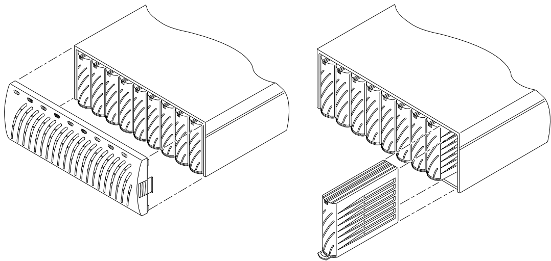
図 11 ディストレーの正面パネルとディスクドライブの取り外し
