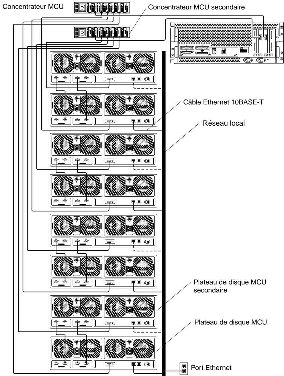
FIGURE 1 Configuration maximale pour Sun StorEdge N8400 Filer
