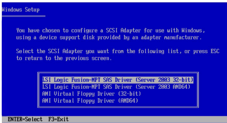
FIGURE 7-4 Écran permettant de sélectionner l'adaptateur SCSI
