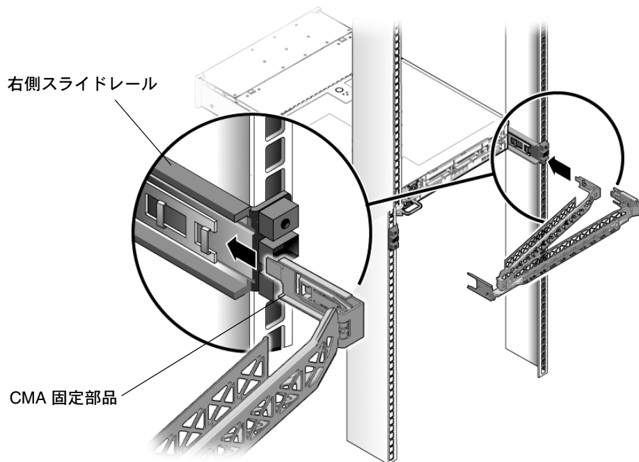
図 2-9 右側スライドレール後部への CMA 固定部品の挿入
