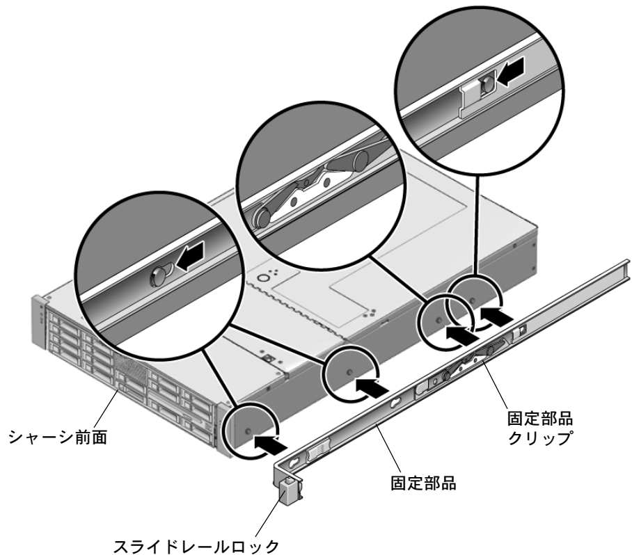
図 2-2 固定部品とサーバーシャーシとの整列
