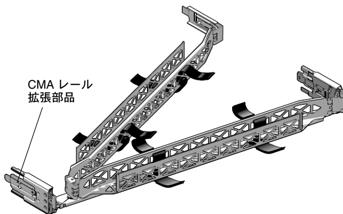
図 2-7 ケーブル管理アーム (CMA)
