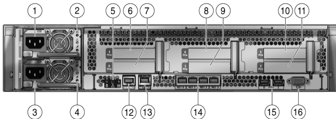
図 1-5 背面パネル
