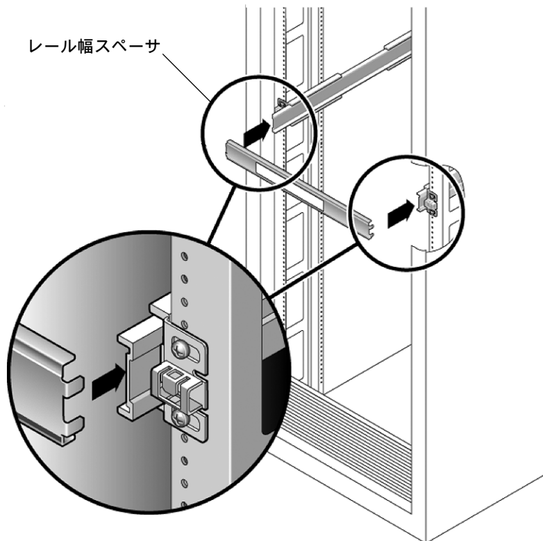
図 2-4 レール幅の設定
