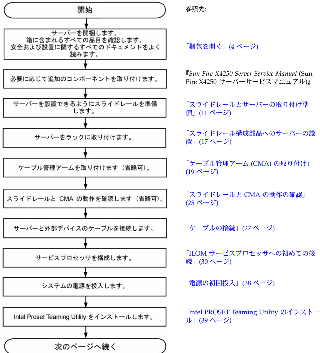
図 1-1 Sun Fire X4250 サーバー設置プロセス (パート 1)
