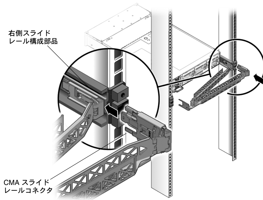
図 2-10 右側スライドレール構成部品の後部への CMA スライドレールコネクタの挿入
