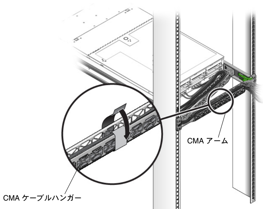
図 2-12 CMA ケーブルストラップの設置
