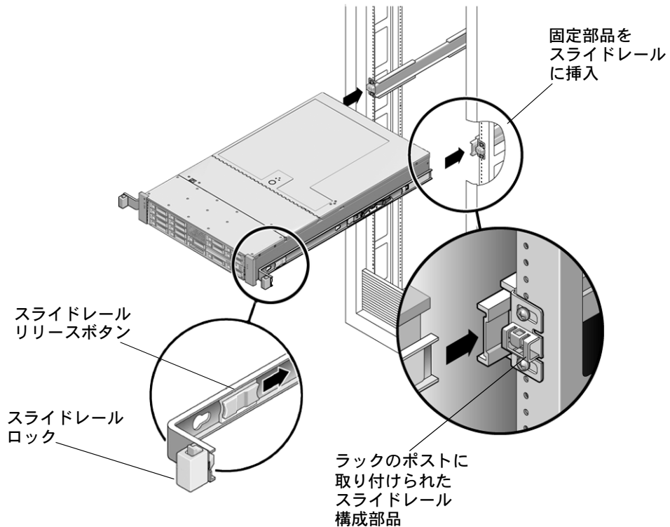
図 2-6 固定部品を取り付けたサーバーのスライドレールへの挿入
