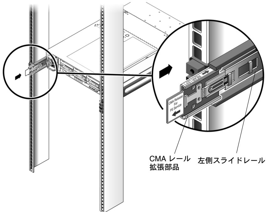
図 2-8 左側スライドレール後部への CMA レール拡張部品の挿入
