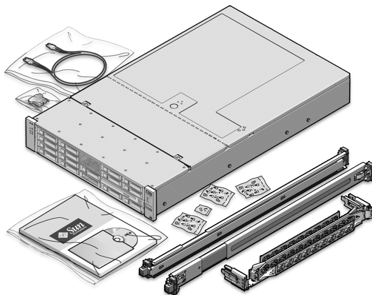
図 1-3 開梱
