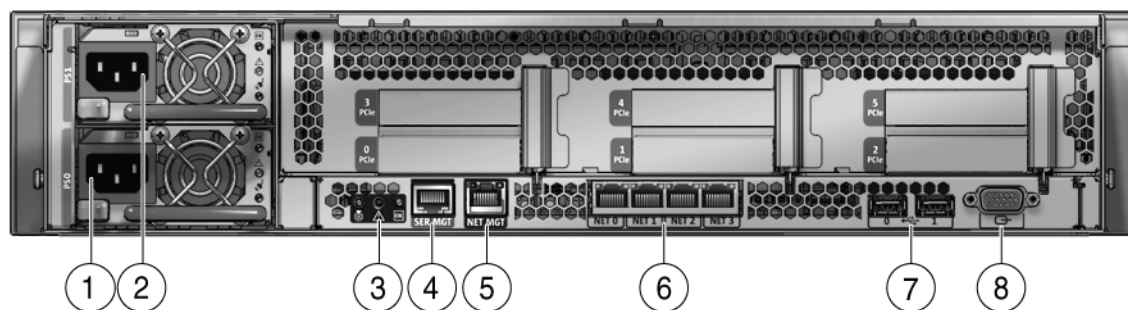
図 3-1 背面パネルコネクタ
