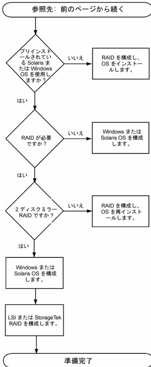
図 1-2 Sun Fire X4250 サーバー設置プロセス (パート 2)
