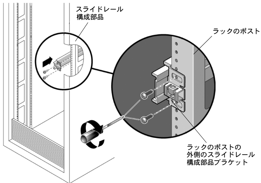
図 2-3 ラックのポストへのスライドレール構成部品の取り付け
