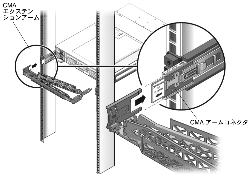
図 2-11 左スライドレールのレール拡張部品コンネクタへの CMA アームの接続
