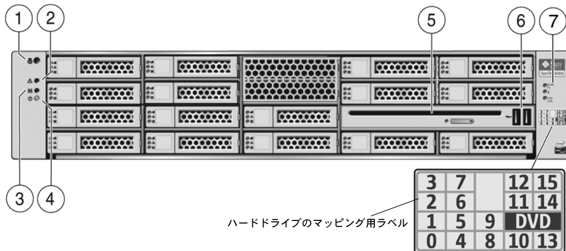
図 1-4 前面パネル
