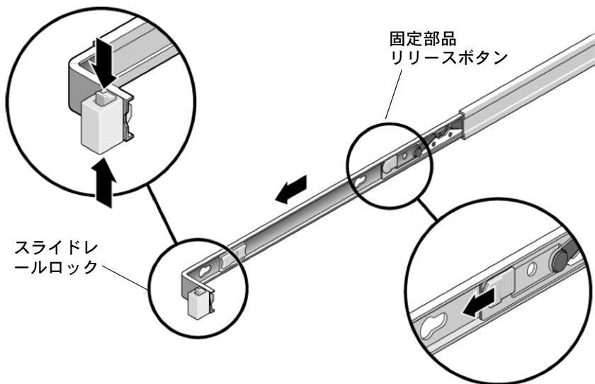
図 2-1 設置前のボルト止めスライドレールの分解
