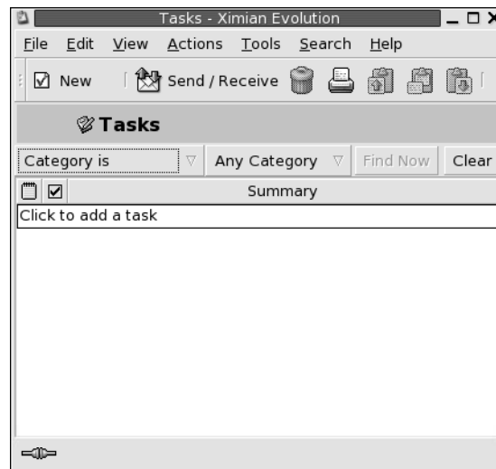
ABBILDUNG 7-1 Typisches Aufgabenfenster
