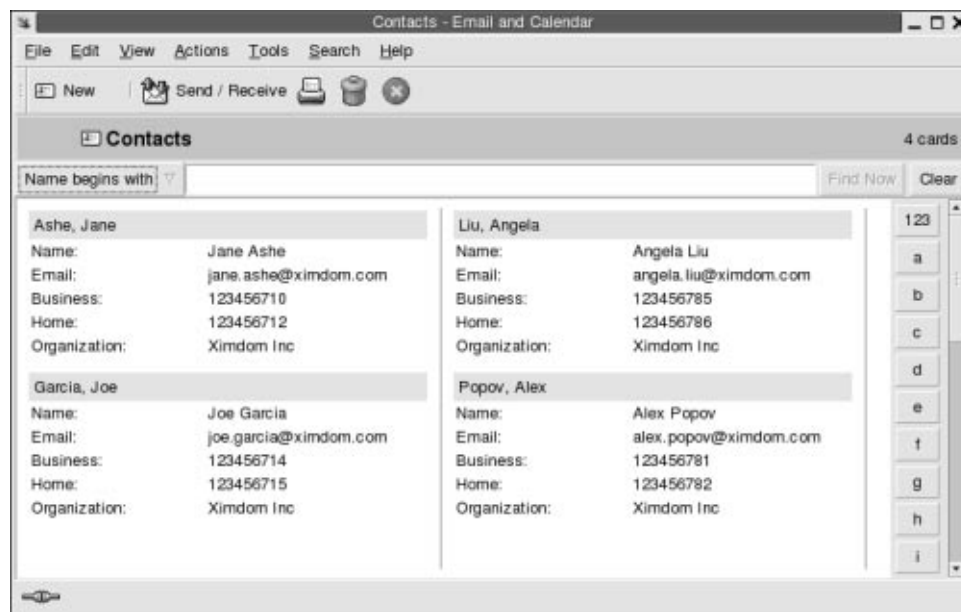
ABBILDUNG 8-1 Typisches Kontaktfenster
