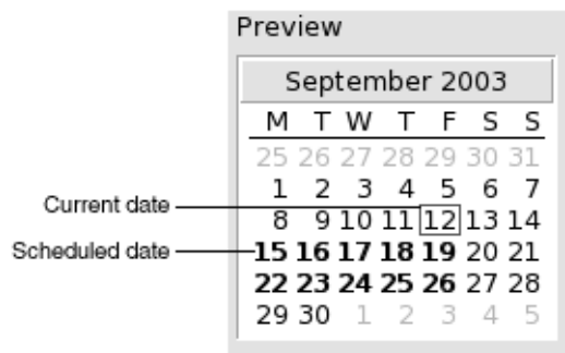
FIGUR 6-2 Typiskt Förhandsgranska-avsnitt
