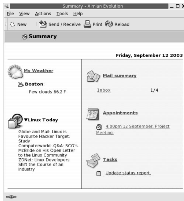
FIGUR 3-1 Typiskt sammanfattningsfönster
