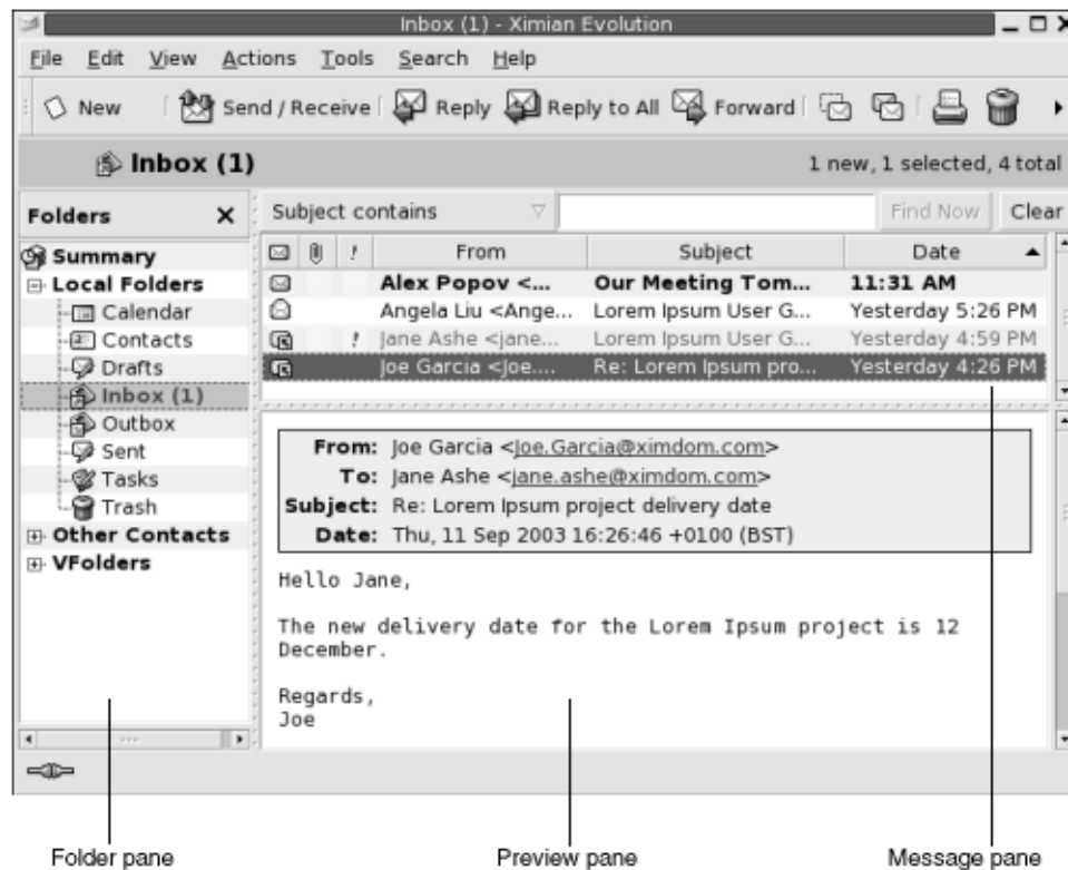
FIGUR 4-1 Typiskt e-postfönster
