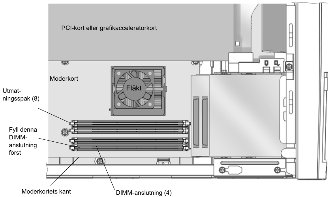
FIGUR 4-6 Installationsordning för DIMM:ar (vy av arbetsstation ovanifrån med höljet borttaget)
