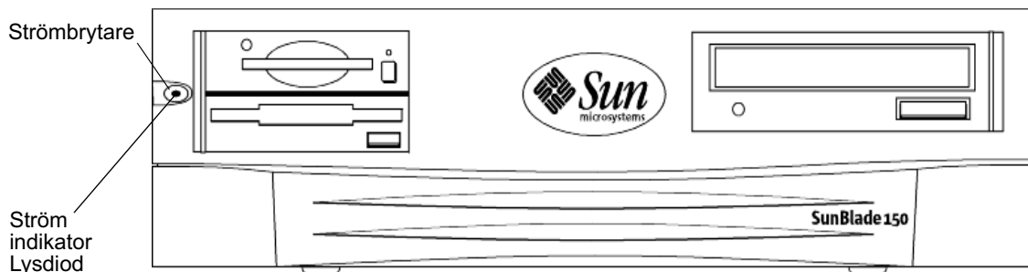
FIGUR 4-1 Placering av strömbrytarens och strömindikeringens lysdioder
