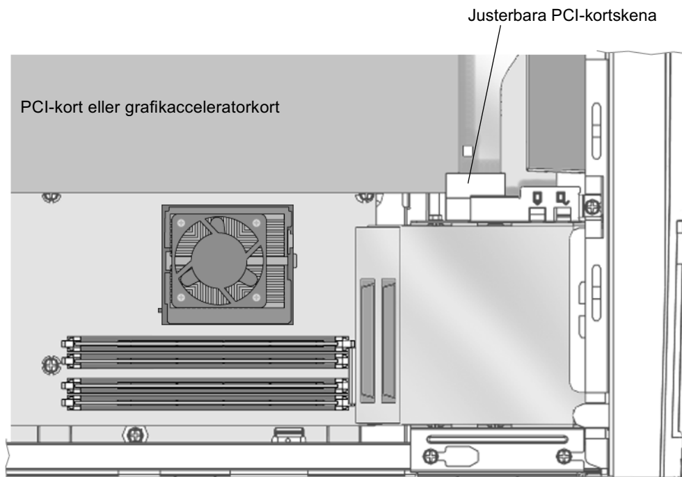
FIGUR 4-9 PCI-kortskenor
