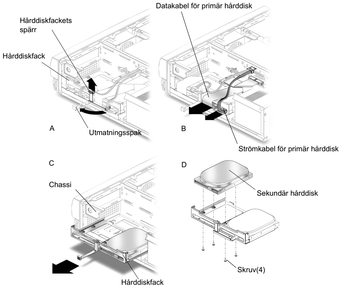
FIGUR 4-11 Installera en sekundär hårdisk
