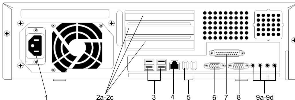
FIGUR 1-4 Översikt, baksida
