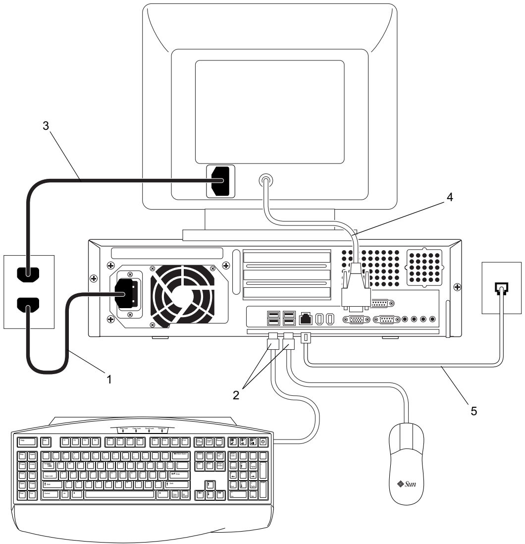
FIGUR 1-6 Koppla ihop arbetsstationen
