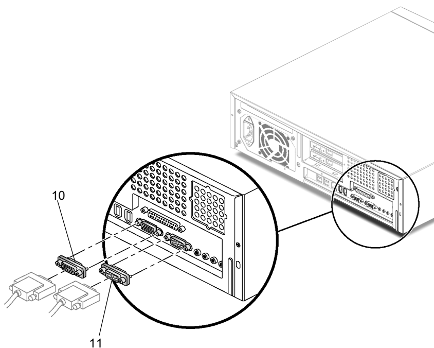
FIGUR 1-5 Förlängningskabel för bildskärms- och serieporten
