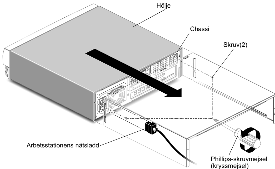
FIGUR 4-3 Ta bort arbetsstationens hölje
