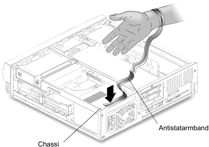
FIGUR 4-4 Fästa antistatarmbandet.
