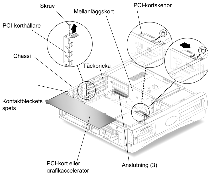
FIGUR 4-8 Installera ett PCI-kort eller en grafikaccelerator
