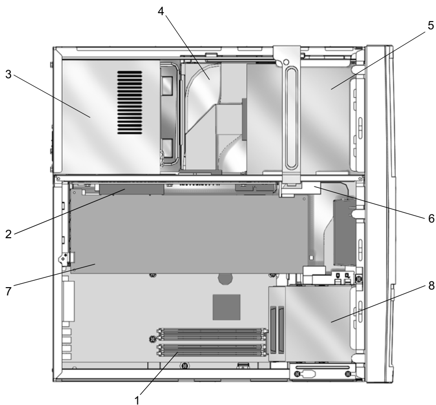
FIGUR 4-5 Arbetsstationens interna layout (sett ovanifrån med borttagen kåpa)
