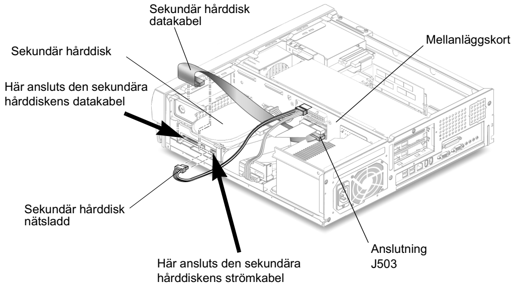
FIGUR 4-12 Ansluta den sekundära hårddiskens kablar
