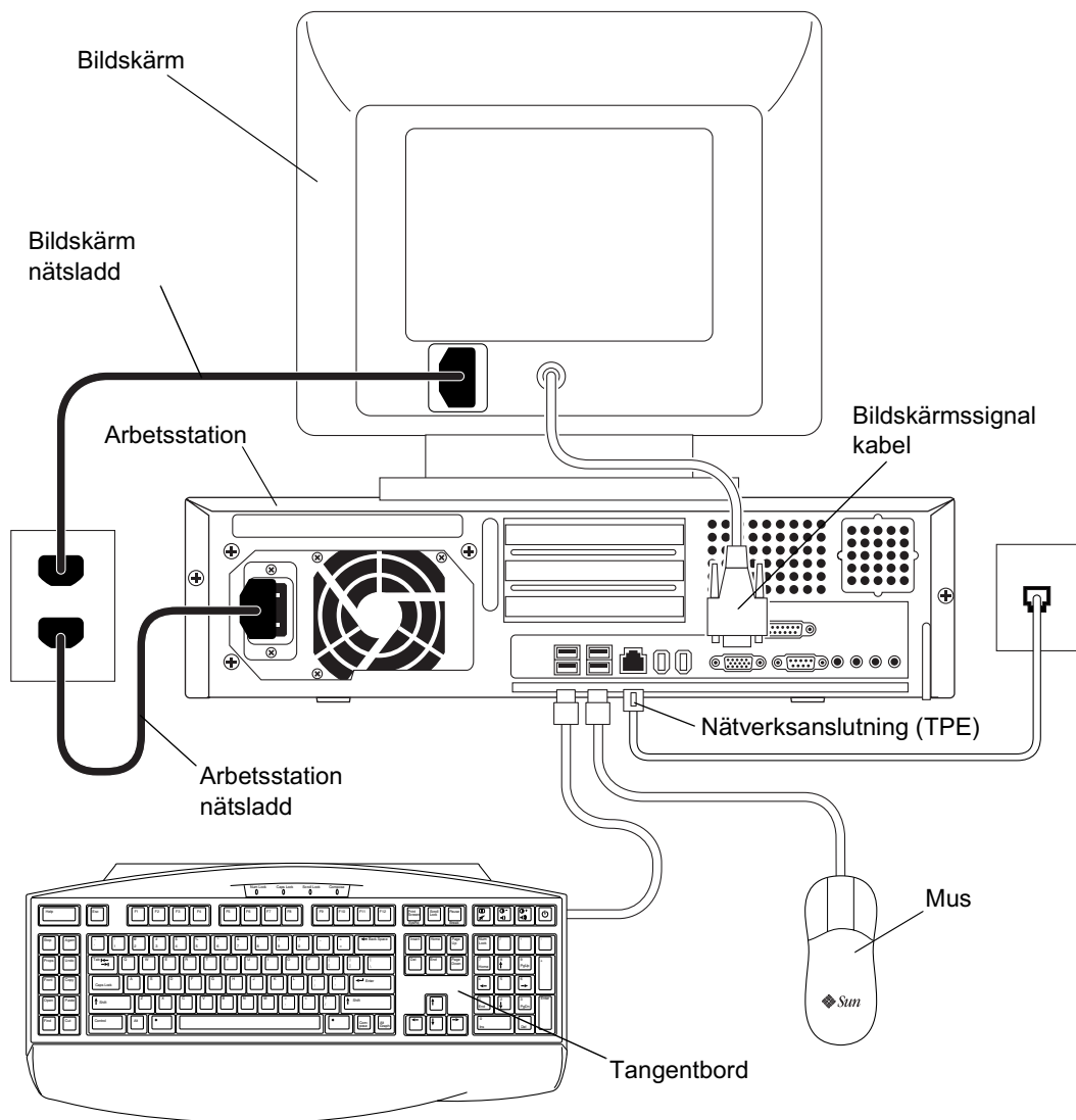
FIGUR 4-2 Koppla bort externa enheter från arbetsstationen
